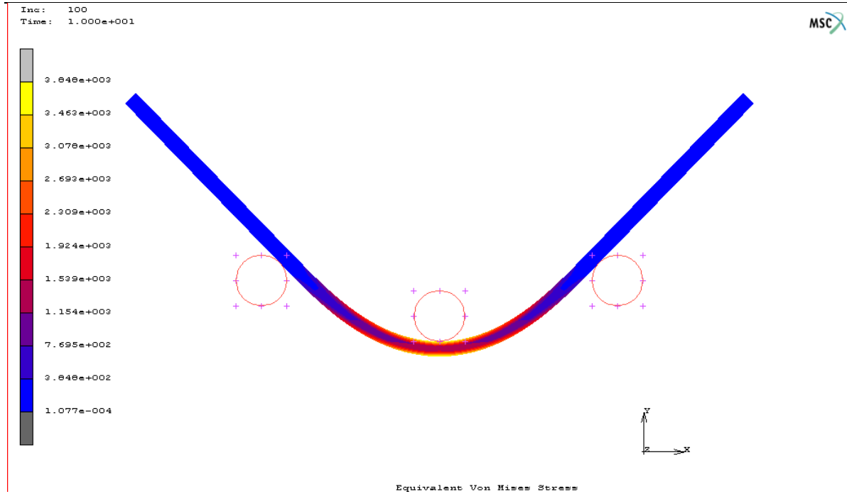
Slika 31. Naprezanja po von Misesu-aluminijski lim, Al99,5
