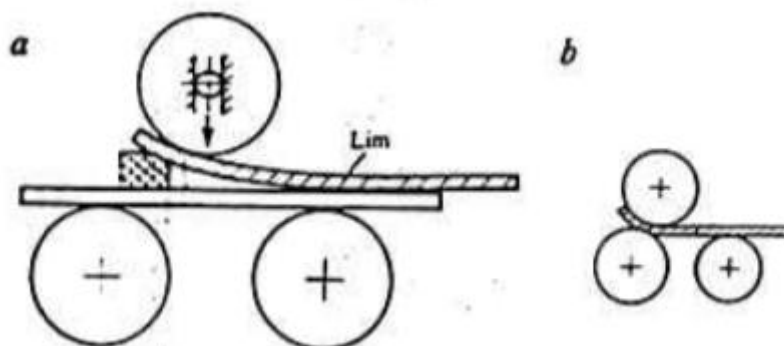
Slika 13. Savijanje u tri točke [16]
