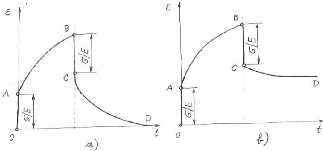
Slika 10. Krivulje puzanja [8]
