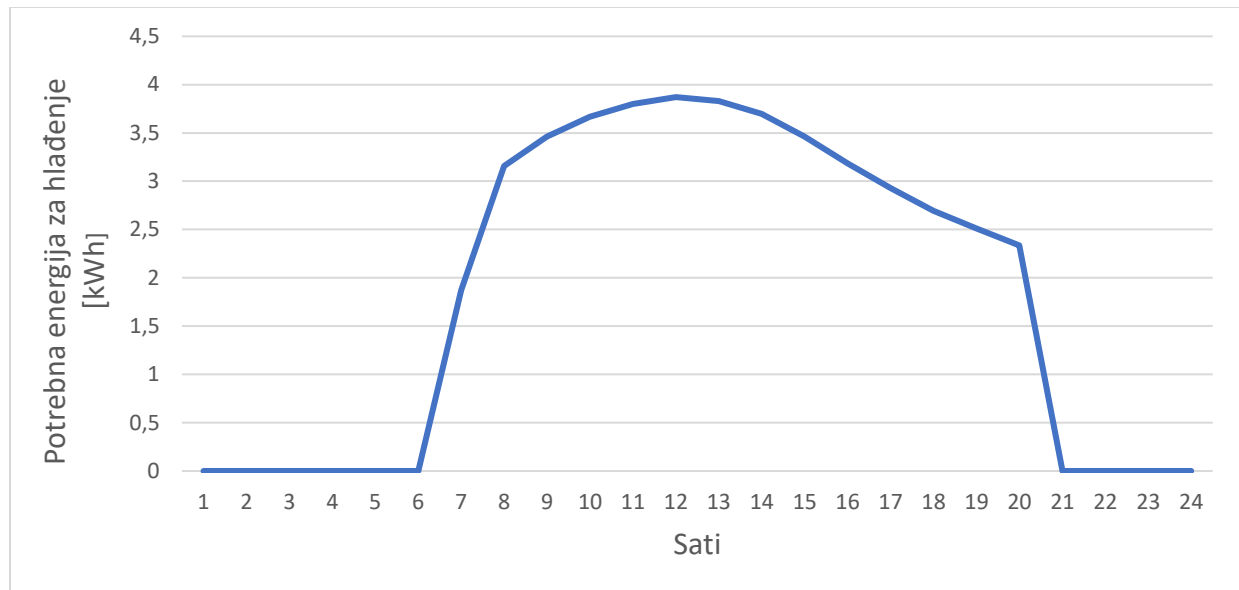
Slika 17. Potrebna energija za hlađenje za karakterističan dan
