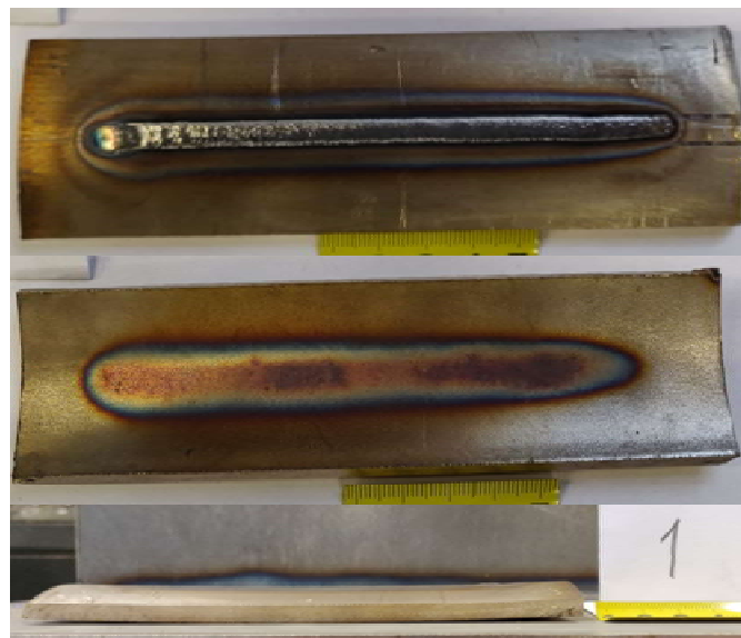
Slika 15. Uzorak 1 ( I = 75 \text{ A} , U = 12,5 \text{ V} )
