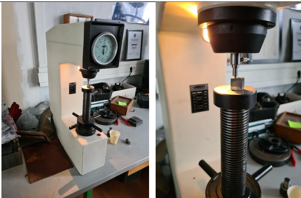
Slika 28. Rockwell indenter „Insize“
