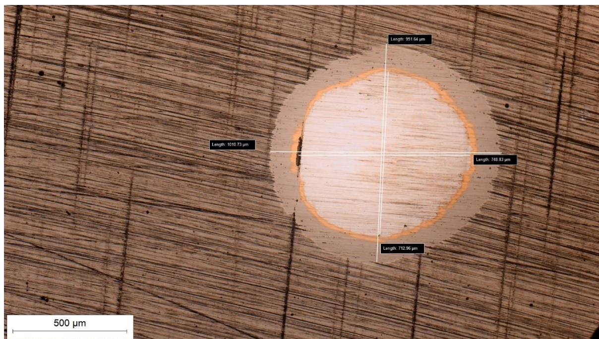
Slika 36. Trag trošenja na čeliku K390 MC snimljen na svjetlosnom mikroskopu nakon ispitivanja debljine prevlake metodom utiskivanja kuglice na uzorku C2 s TiN/TiCN prevlakom
