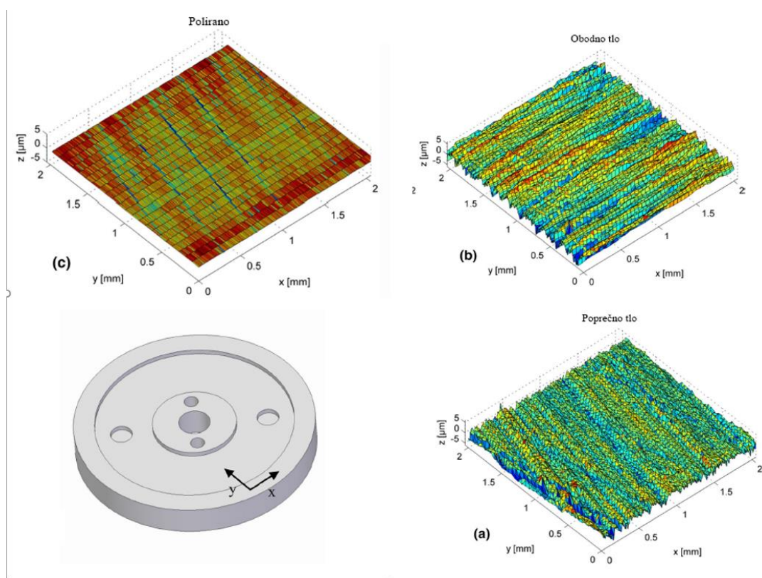
Slika 31. Tri topografije površina: poprečna topografija (a), obodna topografija (b), polirana površina (c) [15].
