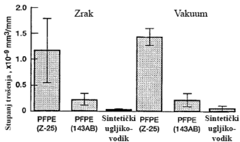
Slika 13. Prikaz stupnjeva trošenja za tri komercijalna maziva u svemirskim ekspedicijama [7].
