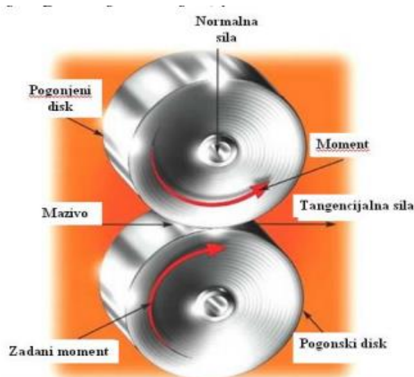
Slika 38. Shema metode dvostrukog diska [6]
