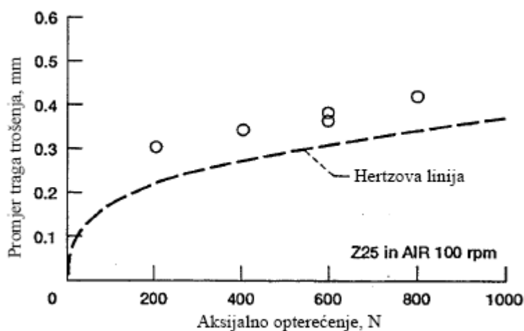
Slika 12. Podaci o trošenju ovisno o aksijalnom opterećenju [7].
