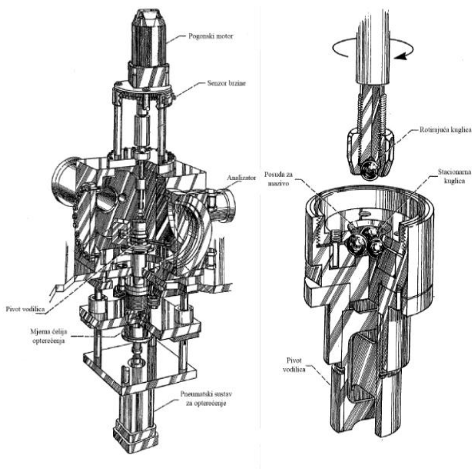
Slika 11. Shema tribouredaja 4 kuglice korištenog u vakuumskom ispitivanju [7].
