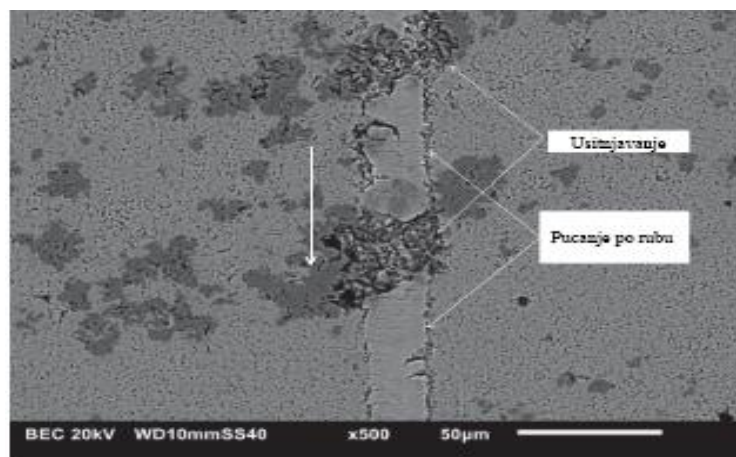
Slika 33. Pucanje po rubu brazde hematita te ustajavanje pukotina getita [14].
