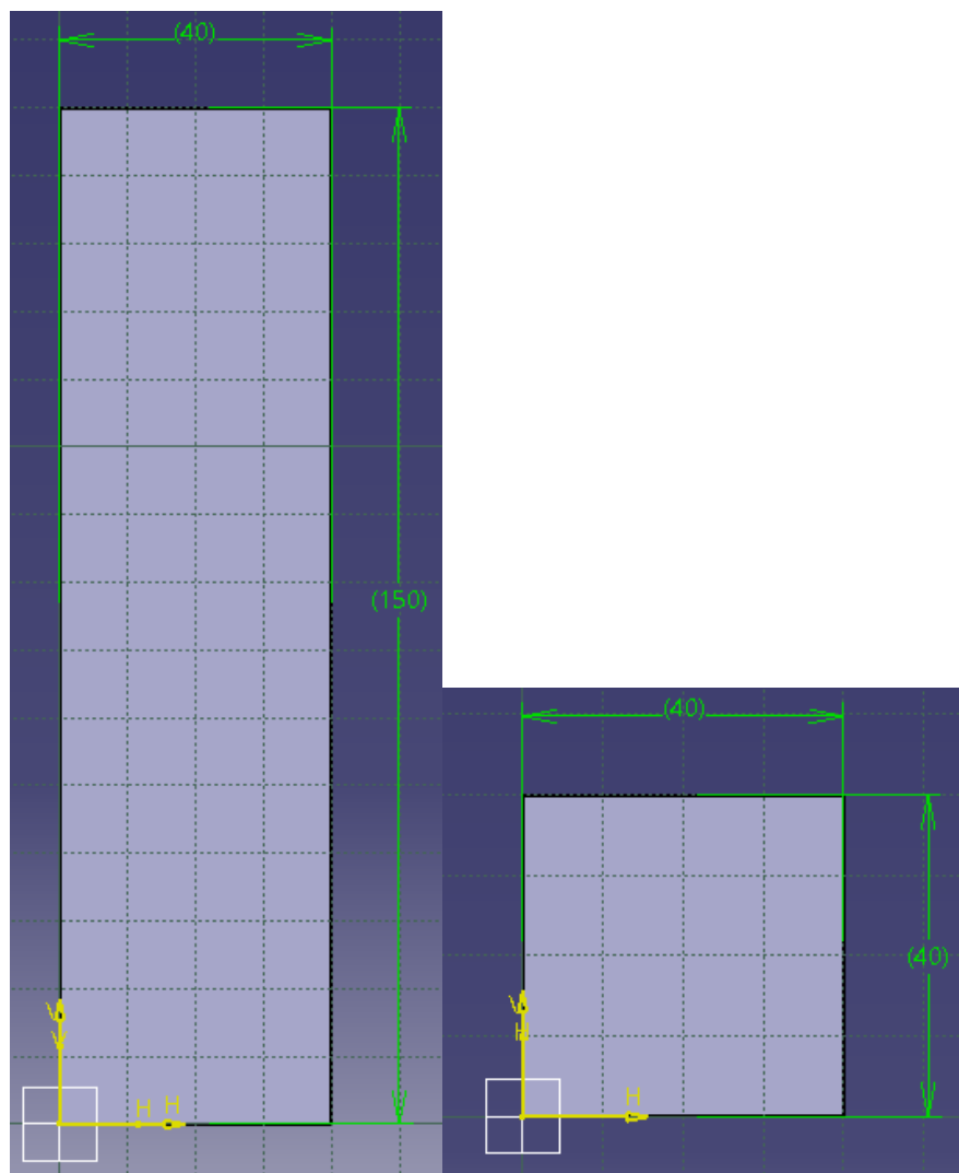
Slika 28. Dimenzije odljevka
