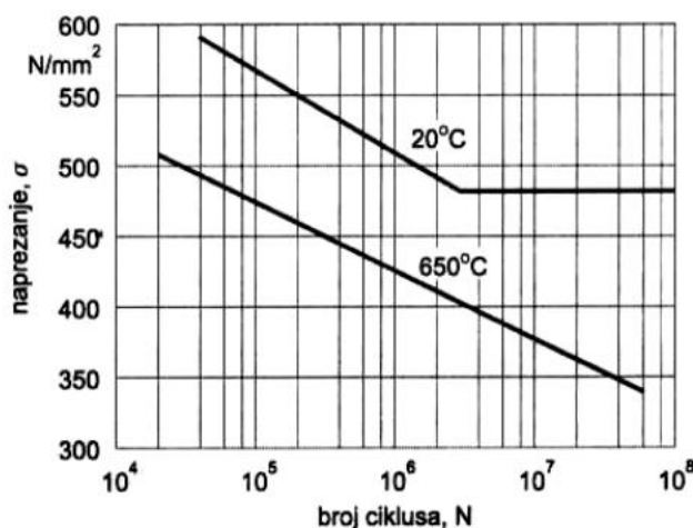
Slika 23. Promjena savojne dinamičke izdržljivosti čelika X10NiCrWTi36-15 s povišenjem temperature [23]
