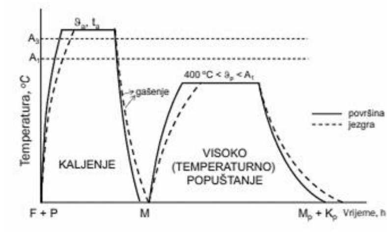
Slika 17. Postupak poboljšavanja [17]
