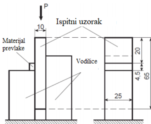
Slika 38. Ispitivanje smicanjem [6]
