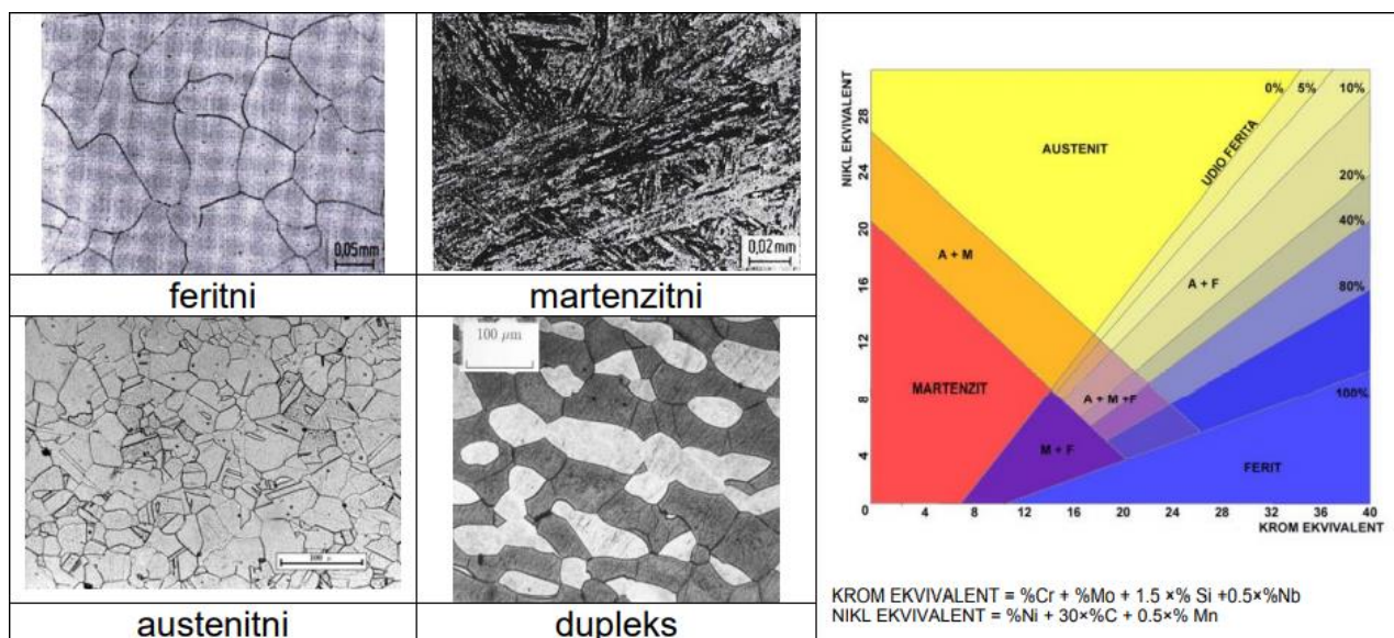
Slika 32. Karakteristične mikrostrukture pojedinih grupa nehrđajućih čelika i strukturni Schaefflerov dijagram [29]
