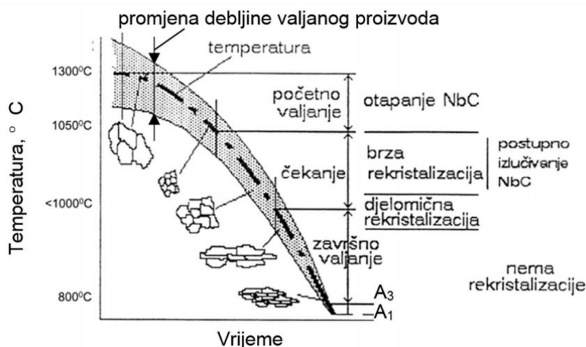
Slika 9. Shematski prikaz zbivanja pri kontroliranom valjanju [7]
