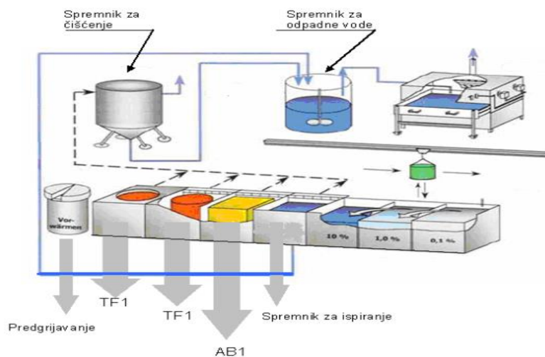
Slika 8. Shematski prikaz postrojenja za nitrokarburiranje s naknadnom oksidacijom u solnim kupkama (TEFIFER QPQ) [10]
