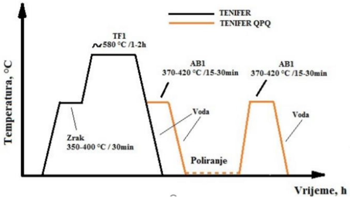
Slika 7. Prikaz TEFIFER i TEFIFER QPQ postupka [9]
