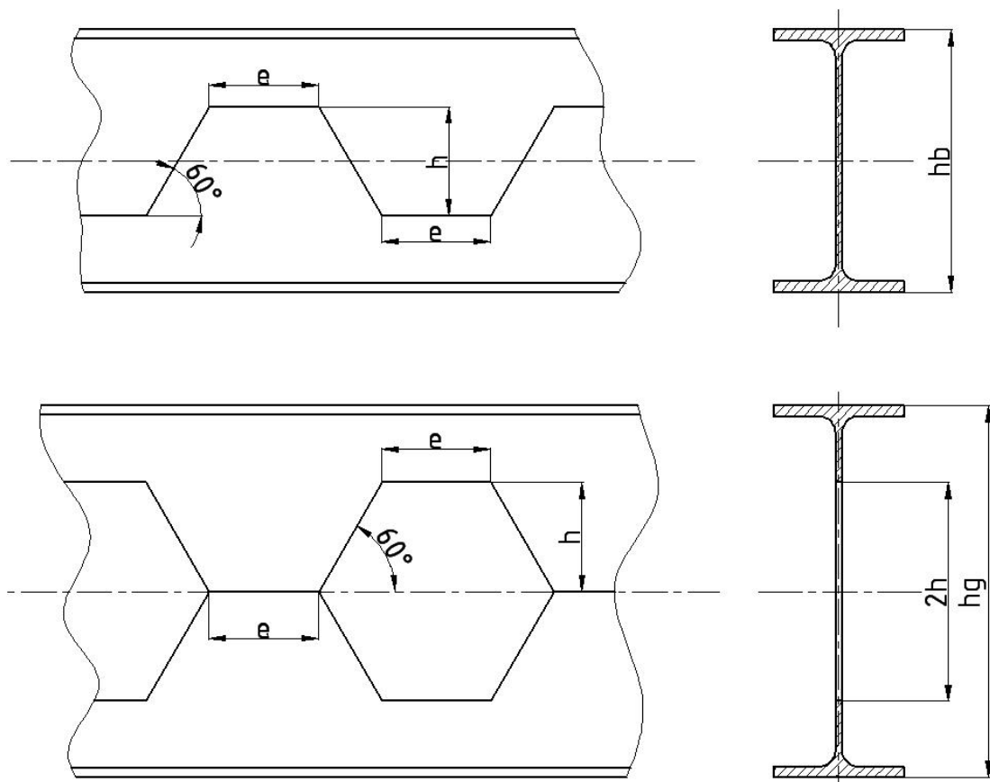
Slika 12. Primjer izrade i dimenzije otvora web-nosača
