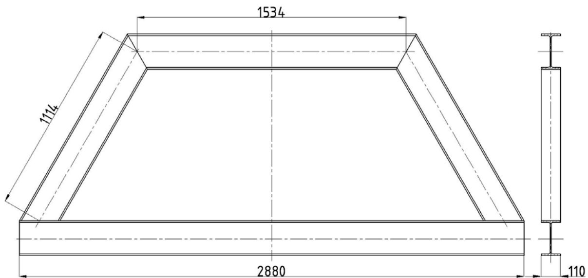
Slika 27. Temeljni nosač
