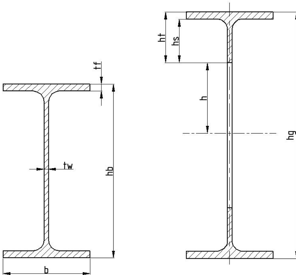
Slika 11. IPE profil i web-nosač izrađen iz tog profila
