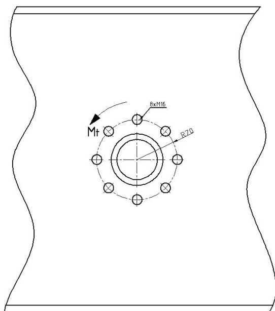
Slika 20. Raspored vijaka
