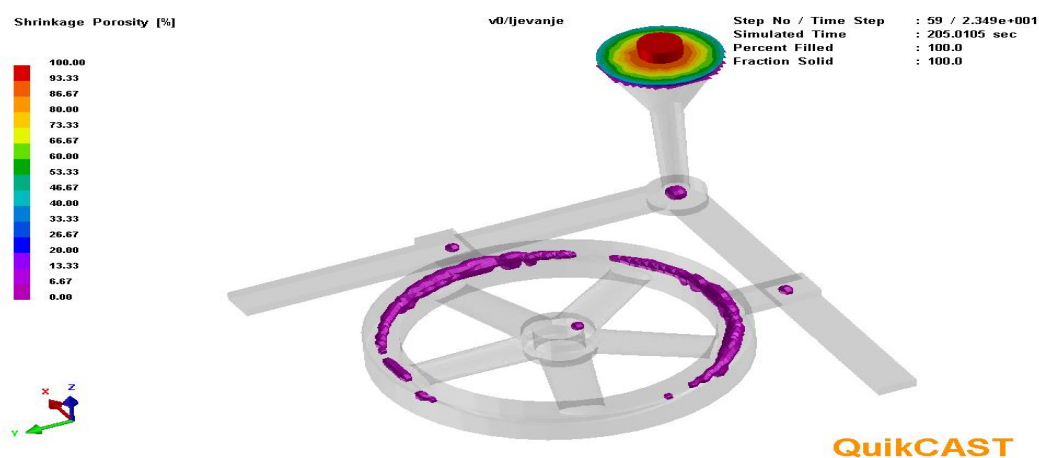
Slika 45. Pojava poroznosti na odljevku bez pojila.
