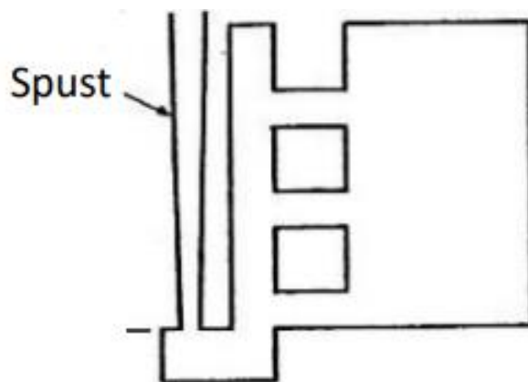
Slika 30. Vertikalni uljevni sustav [1]
