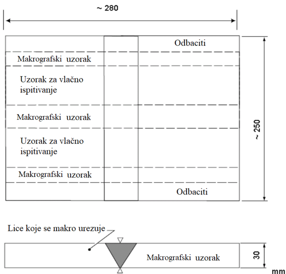
Slika 2.5. Ispitni uzorci [3]
