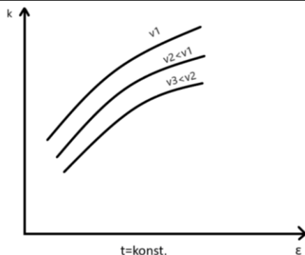
Slika 18. Utjecaj brzine deformacije na specifični deformacijski otpor [13]
