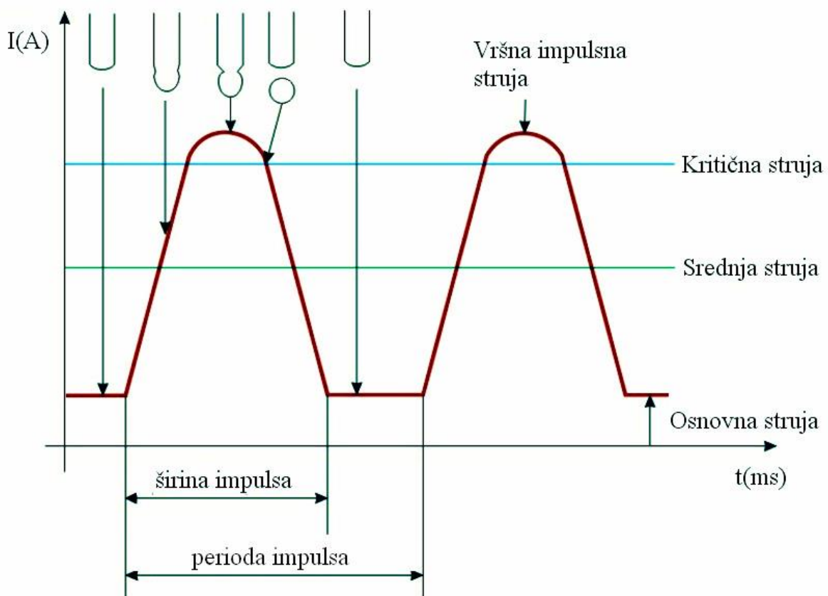
Slika 18. Grafički prikazan impulsnii postupak zavarivanja i otkidanje kapljice [9]
