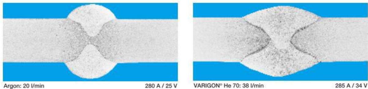
Slika 14. Usporedba utjecaja helija i argona na širinu te profil zavora [21]
