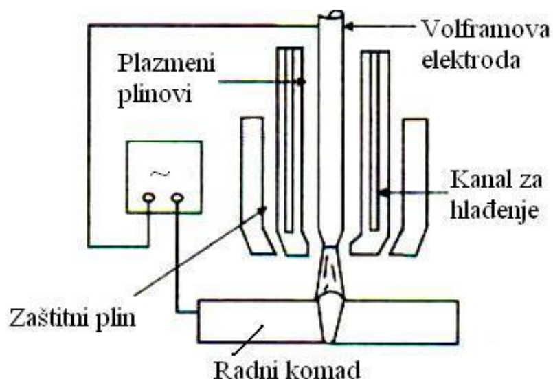
Slika 24. Shematski prikaz plazma postupka zavarivanja [14]
