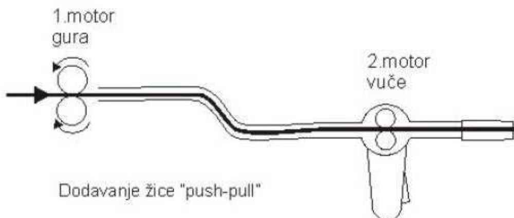
Slika 13. „Push-pull“ sustav dodavanja žice [20]
