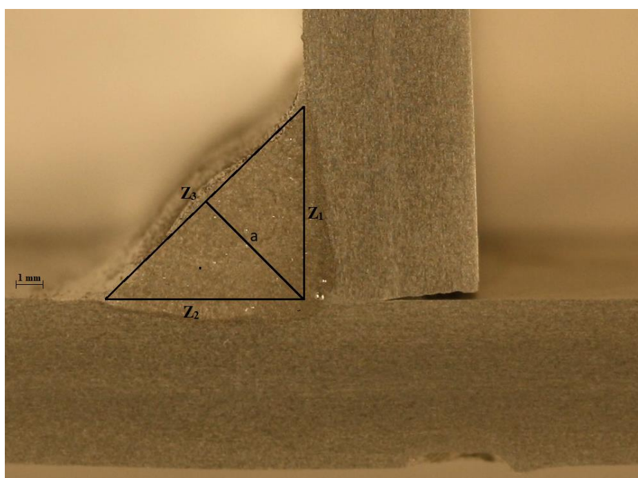
Slika 40. Geometrija zavora
