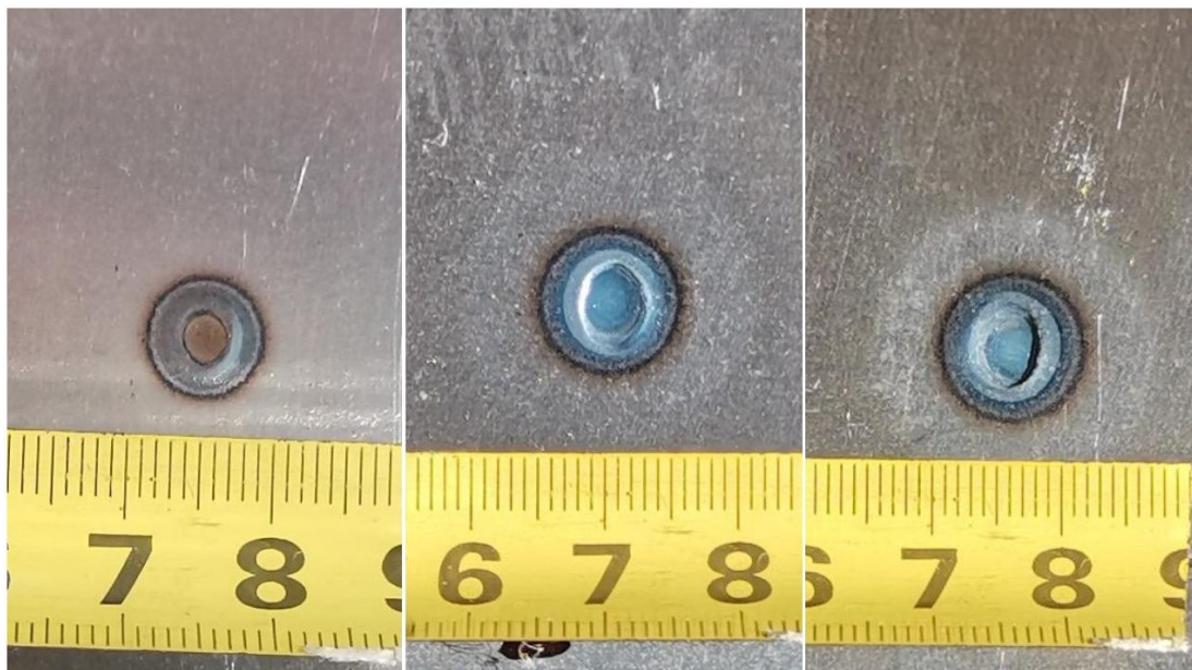
Slika 51 Uvećani prikaz zavara ispitnih uzoraka 4, 5 i 6 (s lijeva na desno)
