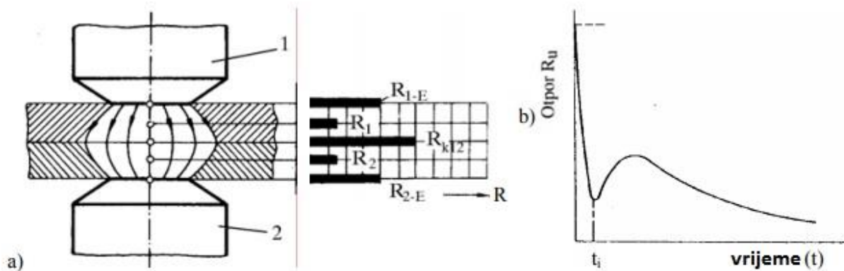
Slika 13 Električni otpori kod točkastog zavarivanja a) početne vrijednosti; b) promjena u vremenu [9]
