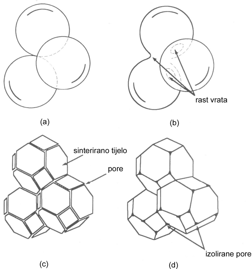
Slika 23. Faze sinteriranja [6]
