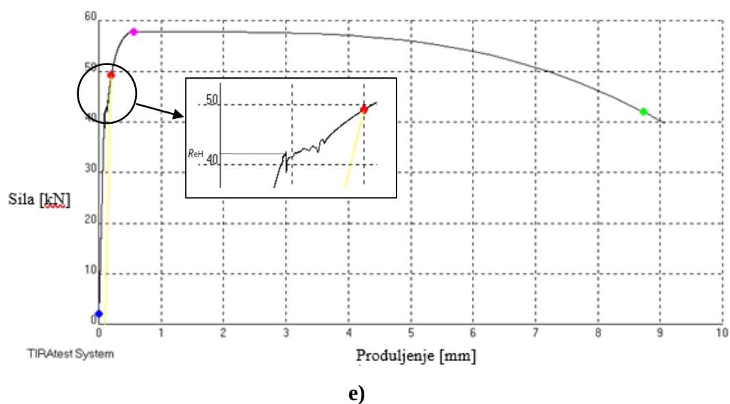
Slika 4.10. Dijagrami sila-produljenje grupa A
