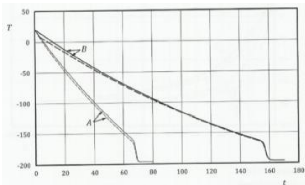
Slika 3.7. Krivulje ohlađivanja ispitnog uzorka u tekućem dušiku na -196 °C [12]
