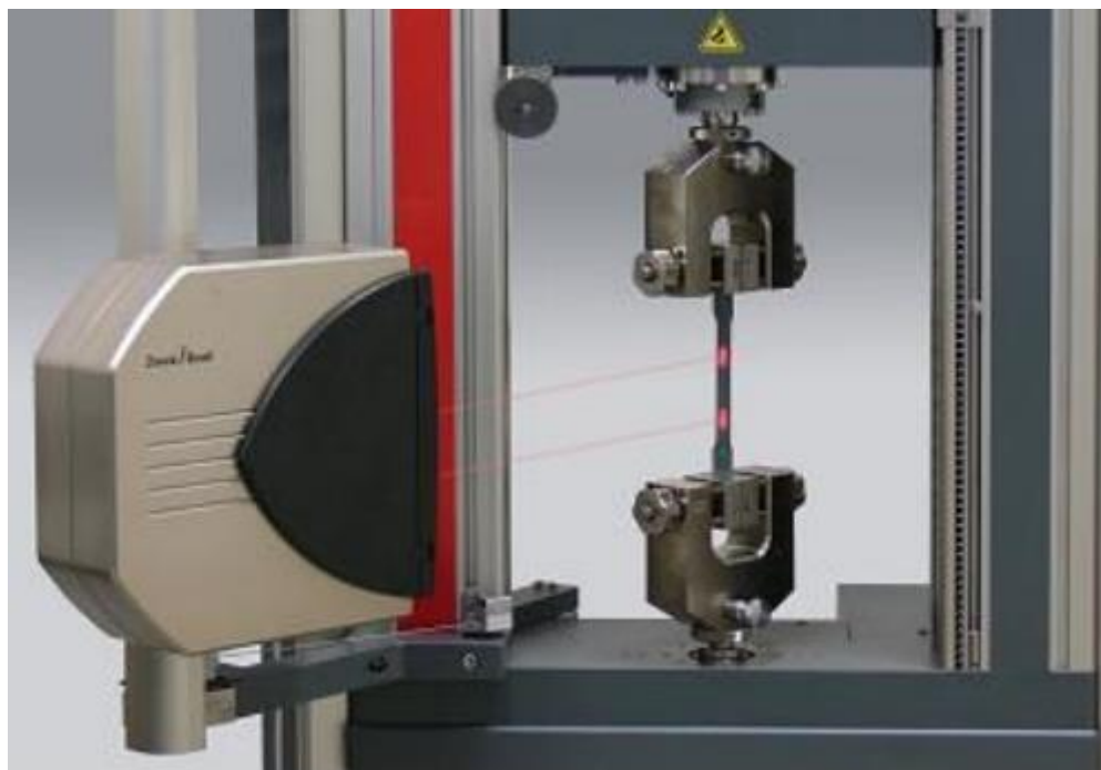
Slika 2.4. Laserski ekstenzometar [6]
