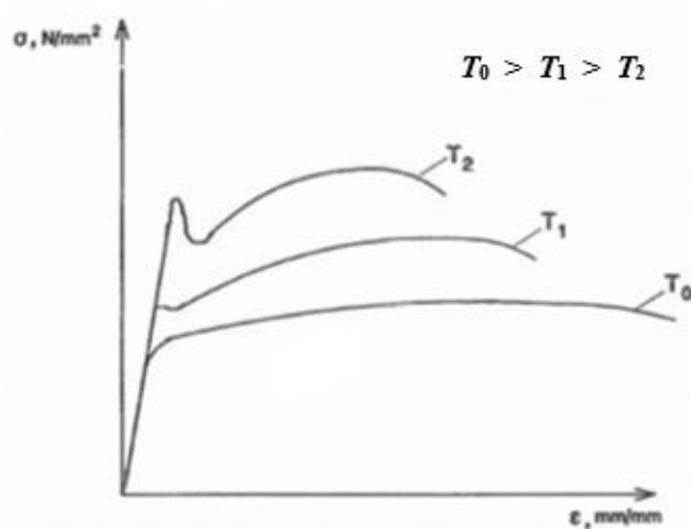
Slika 3.1. Utjecaj snižene temperature na opće konstrukcijske čelike [10]
