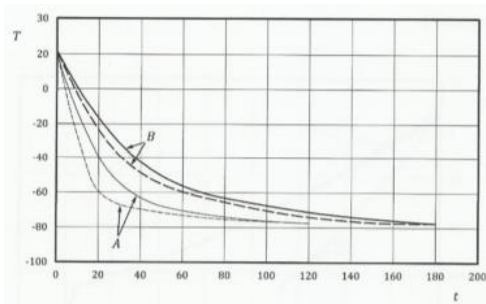
Slika 3.6. Krivulje ohlađivanja ispitnog uzorka u etanolu na -78 °C [12]
