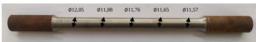
Slika 5.2. Promjeri uzorka
