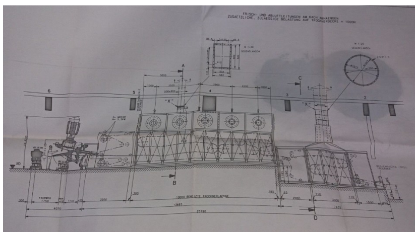
Slika 60. Tehnički crtež sušare - bocort
