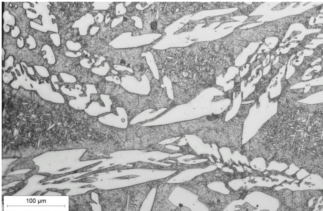
Slika 40. Mikrostruktura toplinski neobrađenog lijeva GX2CrNiMoN 25-6-3, snimljena pri povećanju 200×
