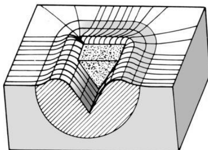
Slika 9. Mikrobraždanje [14]
