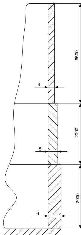
Slika 4.22 Skica odabranih dimenzija za plašt cilindra
