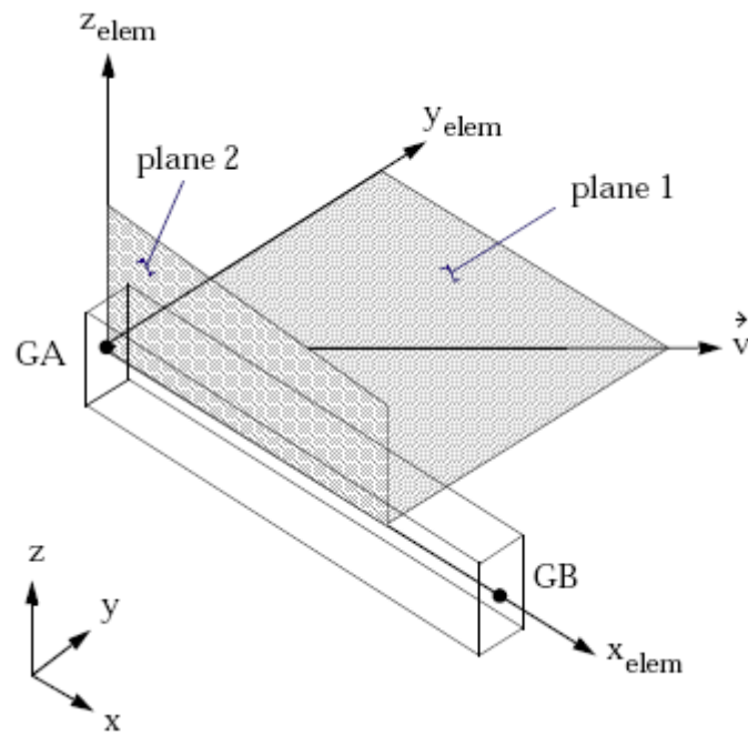
Slika 2.9 Formiranje osi z za CBAR element [2]
