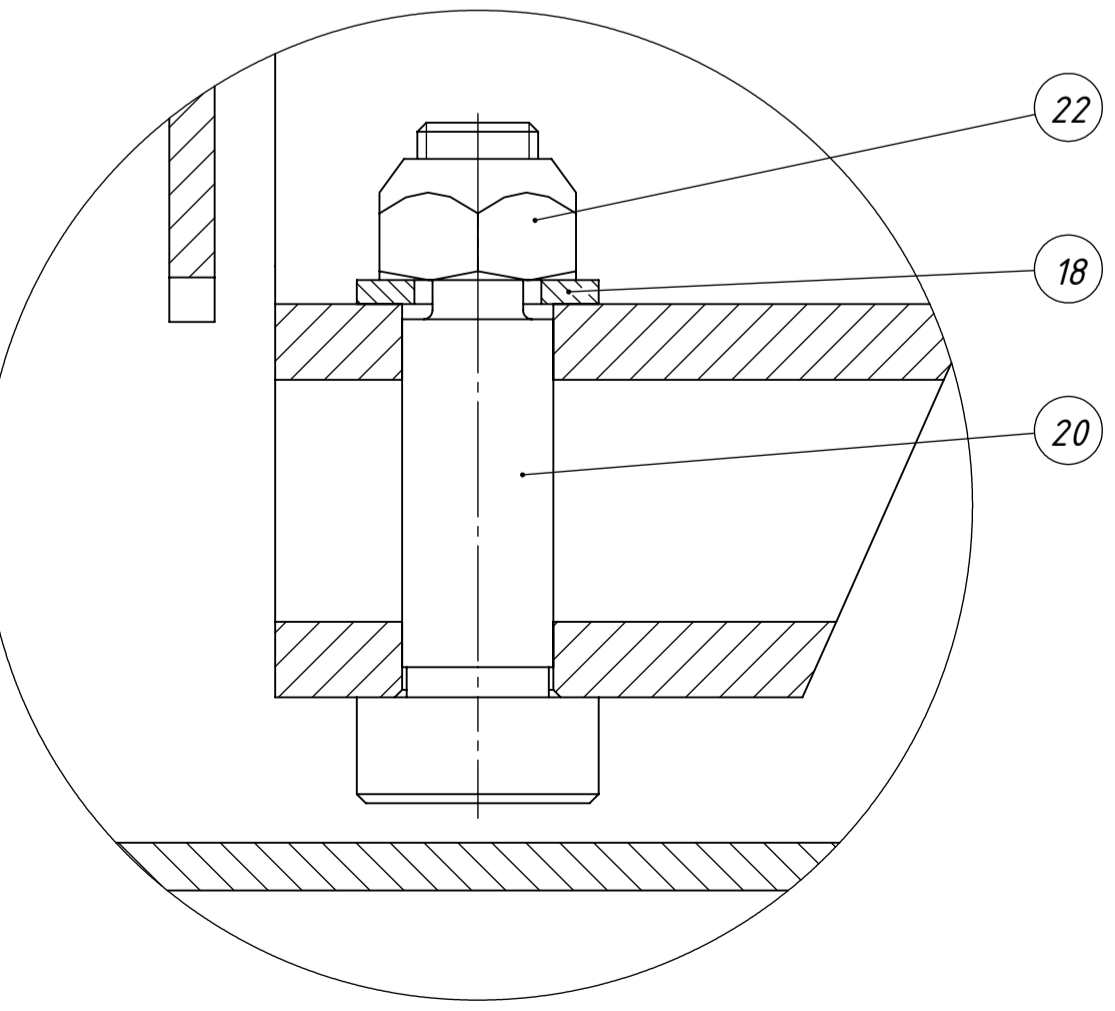
Detalj P Mjerilo M2 : 1
