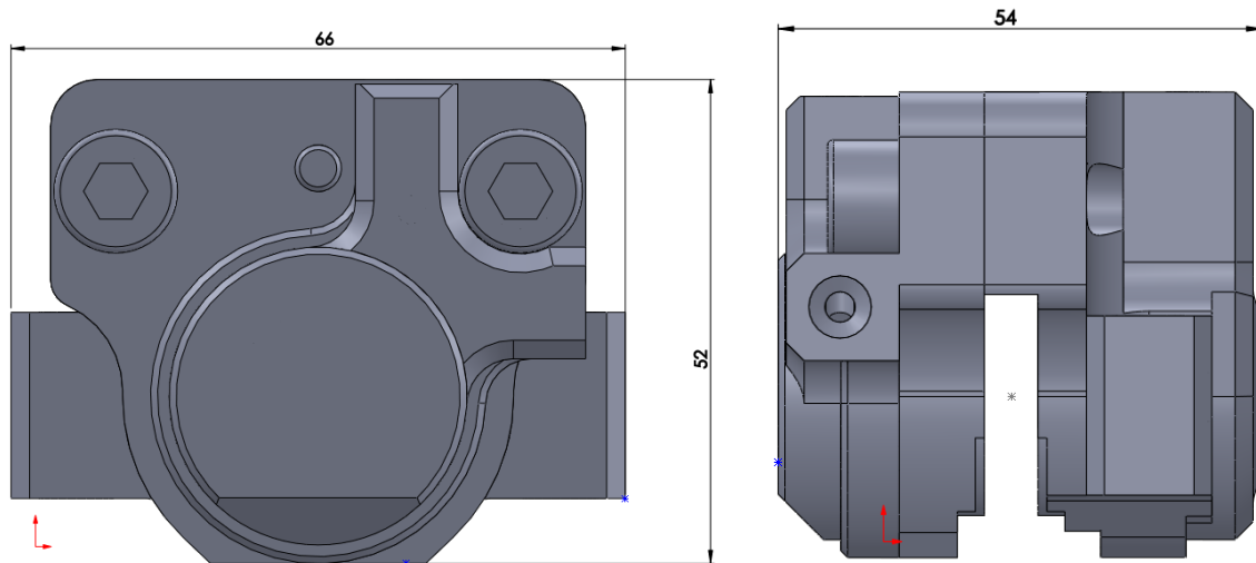
Slika 5. Kočnica
