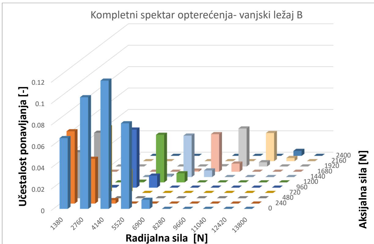
Slika 13. Kompletni spektar opterećenja za vanjski ležaj B
