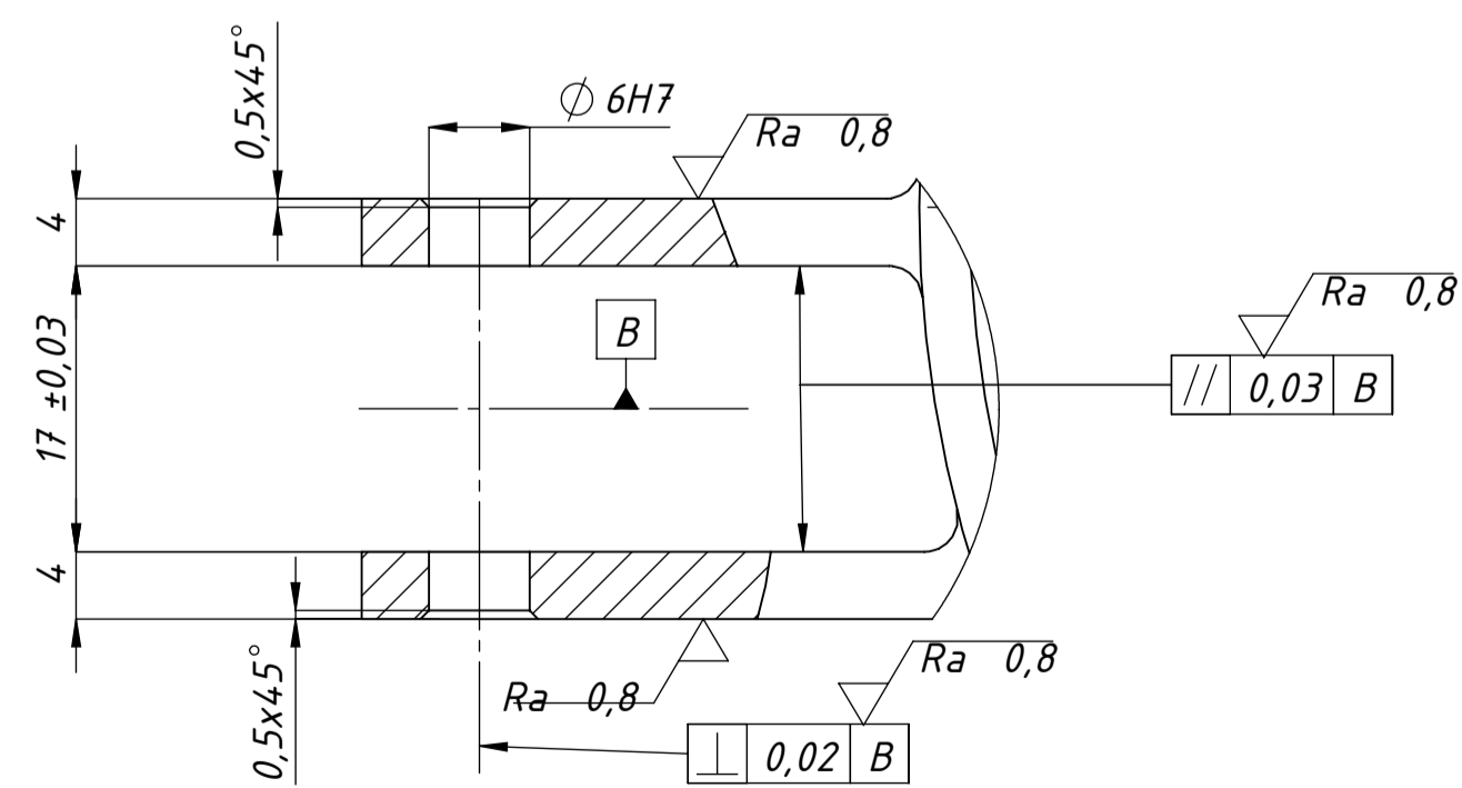
Detalj Z Mjerilo M2 : 1
