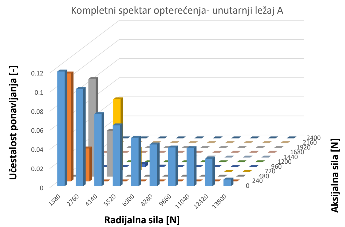
Slika 12. Kompletni spektar opterećenja za unutarnji ležaj A
