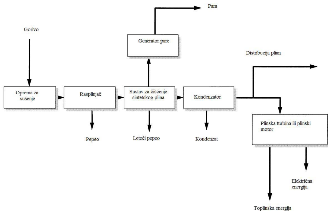
Slika 4.1. Prikaz postrojenja za energetske oporabu komunalnog otpada [12]
