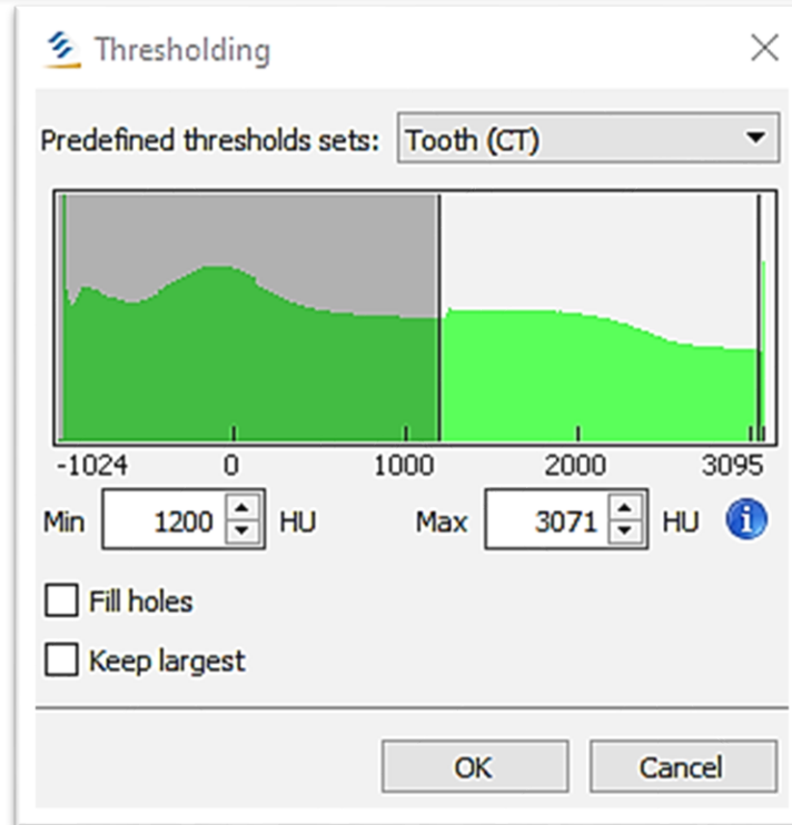
Slika 5.2 Thresholding
