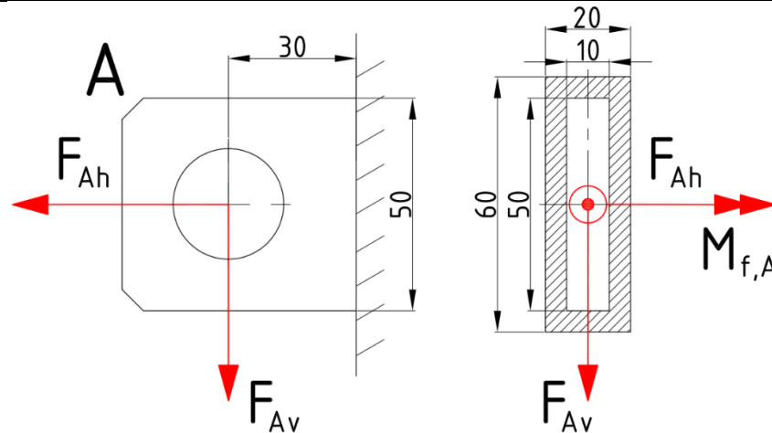
Slika 53. Opterećenje i geometrija zavora ušice u osloncu A
