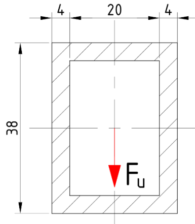
Slika 51. Proračunski presjek zavar a ušice
