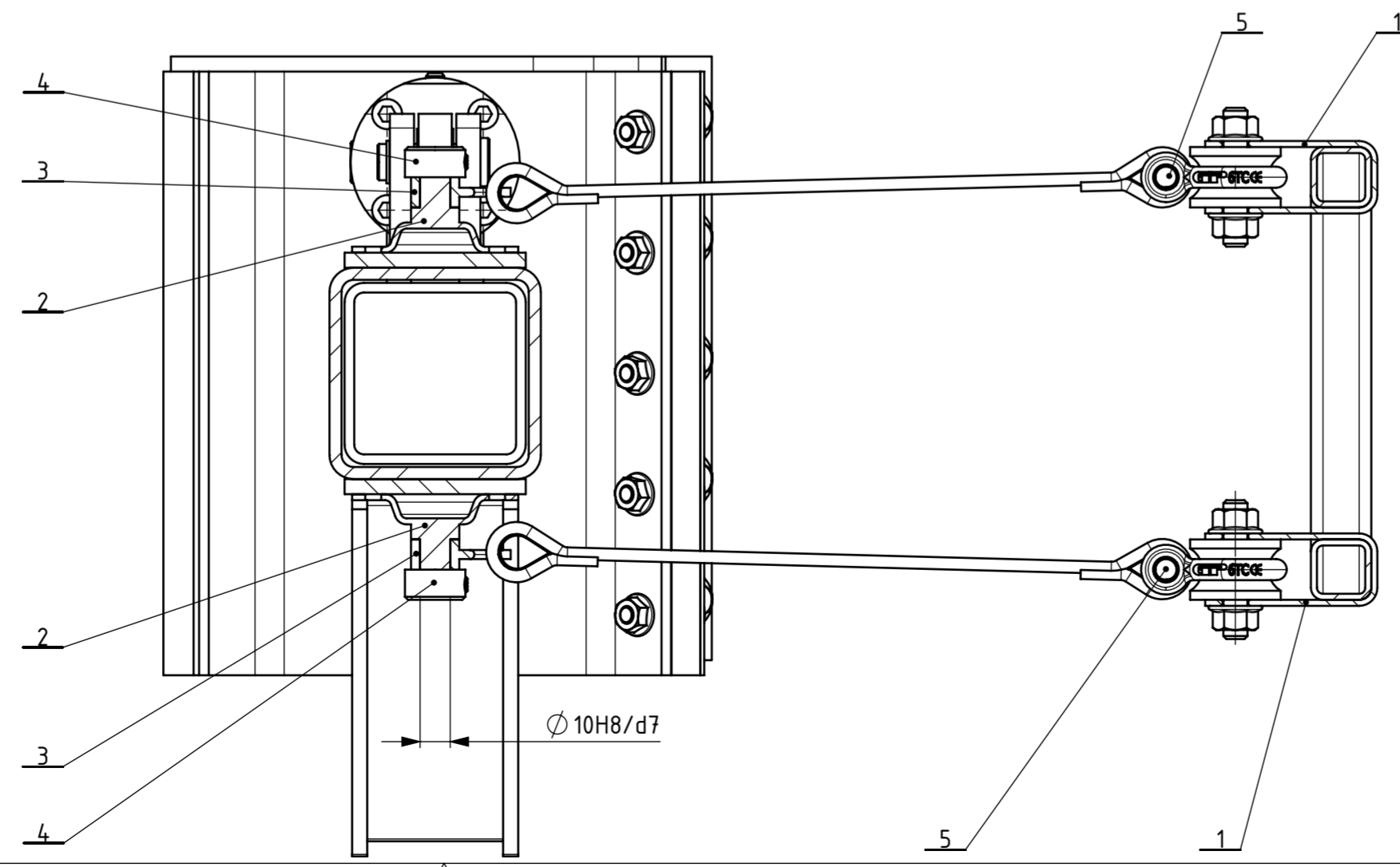
A-A M 1:2
