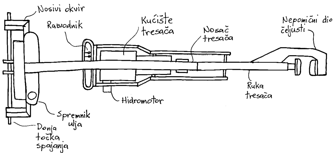
Slika 37. Koncept 3 – tlocrt
