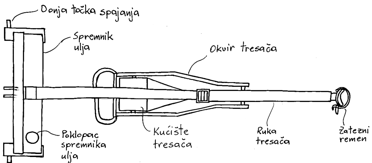
Slika 31. Koncept 1 – flocrt
