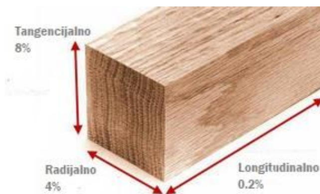
Slika 10. Utjecaj vlage na bubrenje u karakterističnim osima drva [10]
