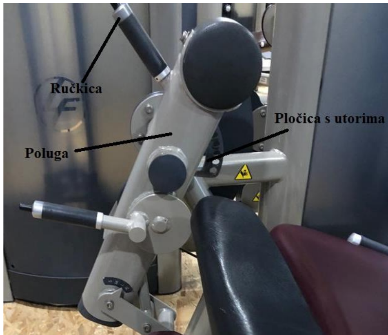
Slika 25. Podesivost poluge
