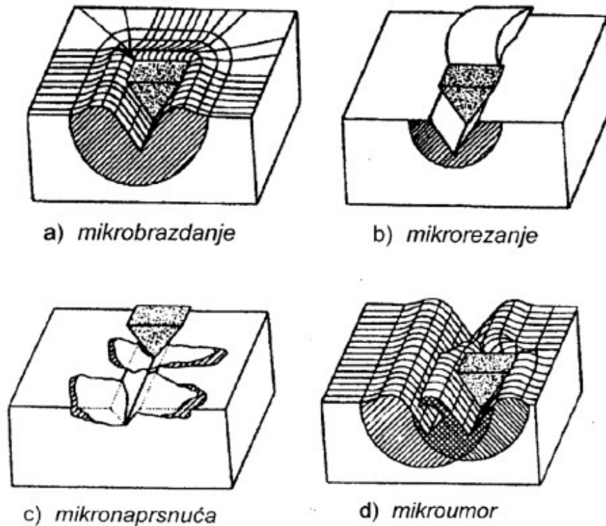
Slika 6.3. Shematski prikaz mikromehanizama trošenja materijala [15]
