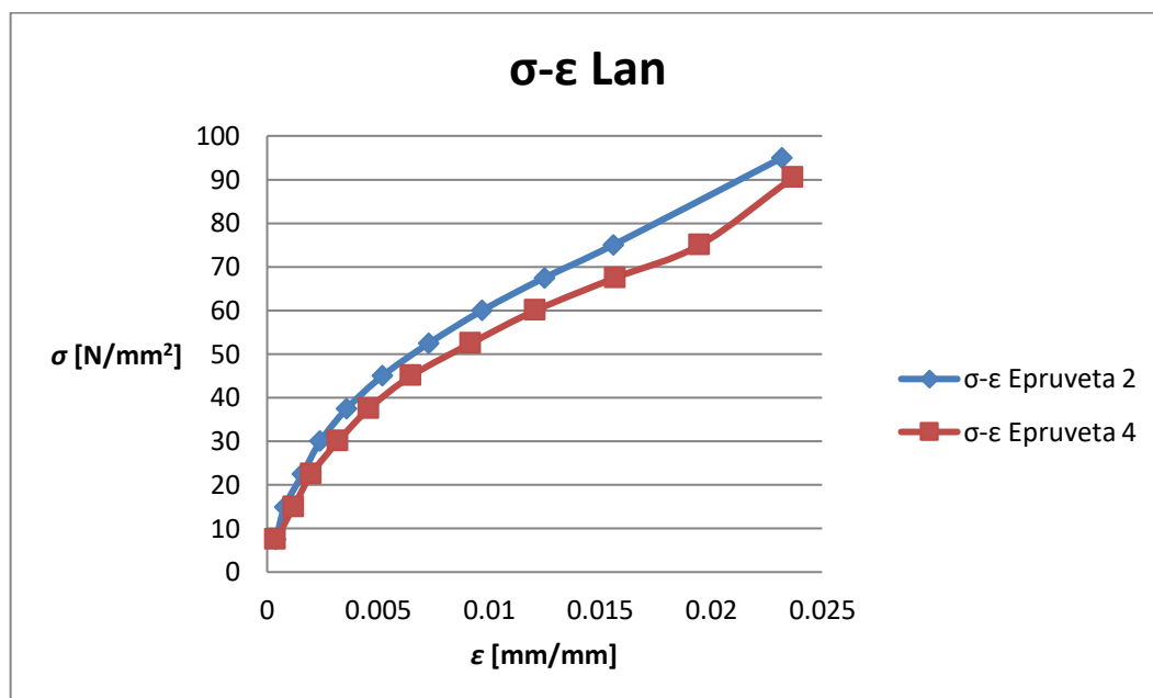
Slika 5.18. Dijagram „naprežanje - istežanje“ za lan
