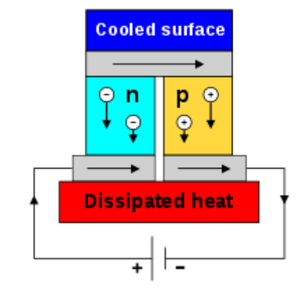
Slika 5. Peltierov (termoelektrični) efekt
