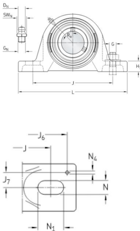
Slika 44. Montažne mjere ležajnog mjesta SKF 35 TF
