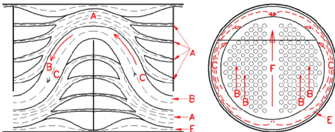
Slika 7. Putanje strujanja unutar plašta izmjenjivača topline s pregradama [10]
