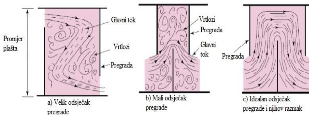
Slika 8. Utjecaj malog i velikog odsječka pregrade [8]
