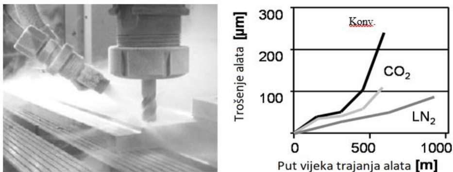
Slika 4. Kriogena obrada [1]
