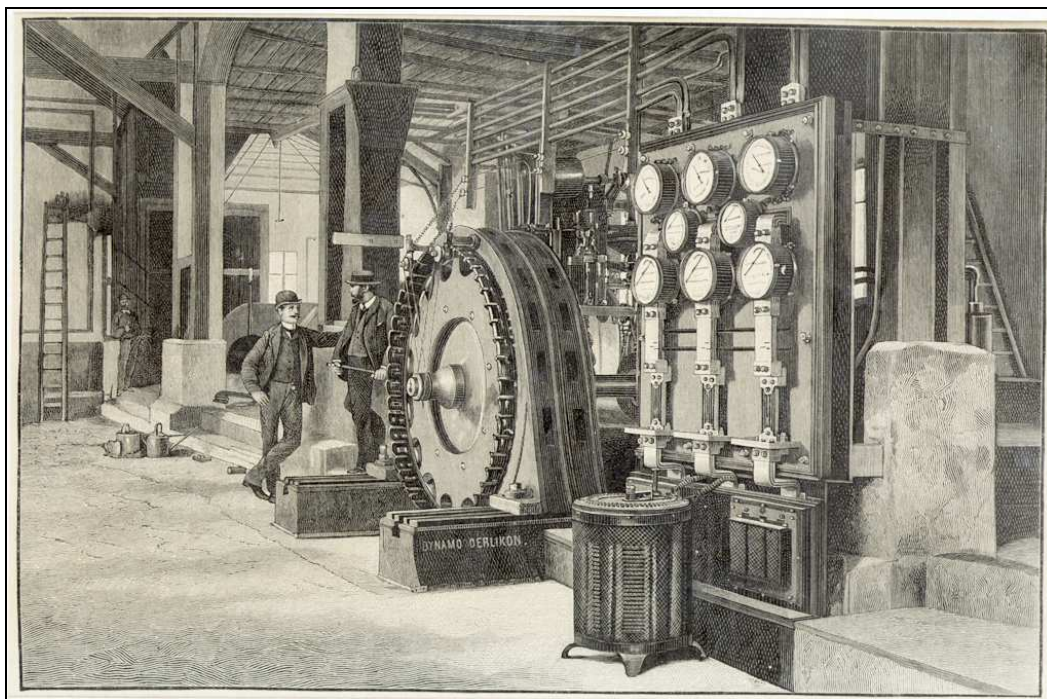
Slika 1-2: Unutrašnjost hidroelektrane na rijeci Neckar (1891. god) – [1]
