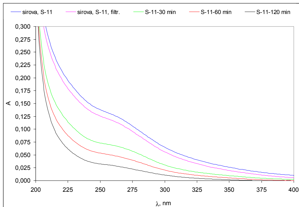
Slika 57. Promjena UV spektra organskih tvari površinske vode u točkama 30, 60 i 120 minuta trajanja eksperimenta, nakon filtracije na 0,45 \mu\text{m} membrani
