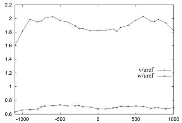
v/u_{ref} ; w/u_{ref}
