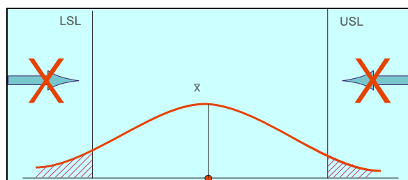
Slika br. 4.8 – Loša kvaliteta – proces nije sposoban
