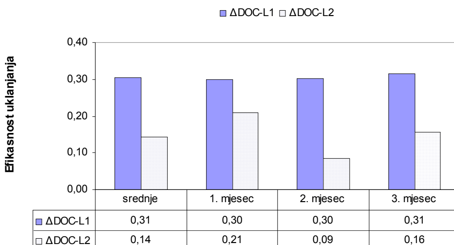
Slika 70. Utjecaj ozonizacije na pad sadržaja otopljenog organskog ugljika (DOC) DOC mjereno tijekom tri mjeseca na liniji L1 i L2 a,b,c
