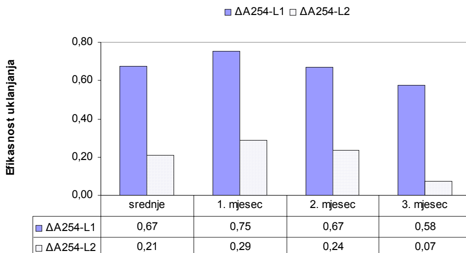
Slika 69. Utjecaj ozonizacije na pad apsorbancije kod 254 nm Redukcija A_{254} mjerena tijekom tri mjeseca na liniji L1 i L2 a,b,c
