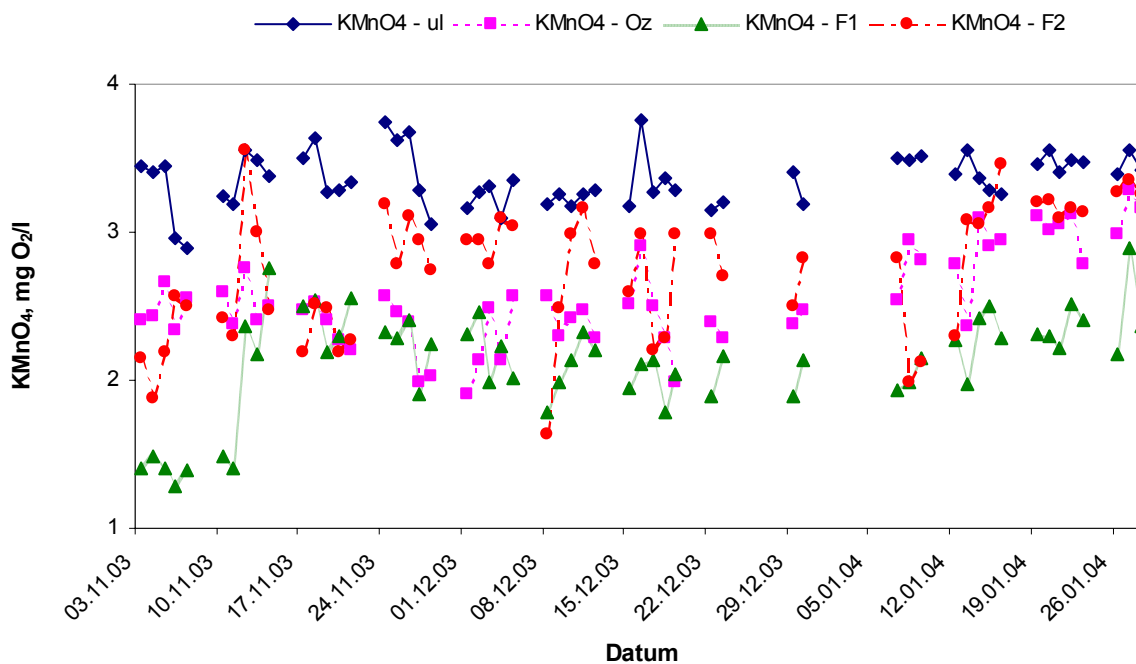
Slika 75. Promjena utroška KMnO_4 mjenog na četiri karakteristična mjesta pilot uređaja tijekom tromjesečnog pilotiranja
