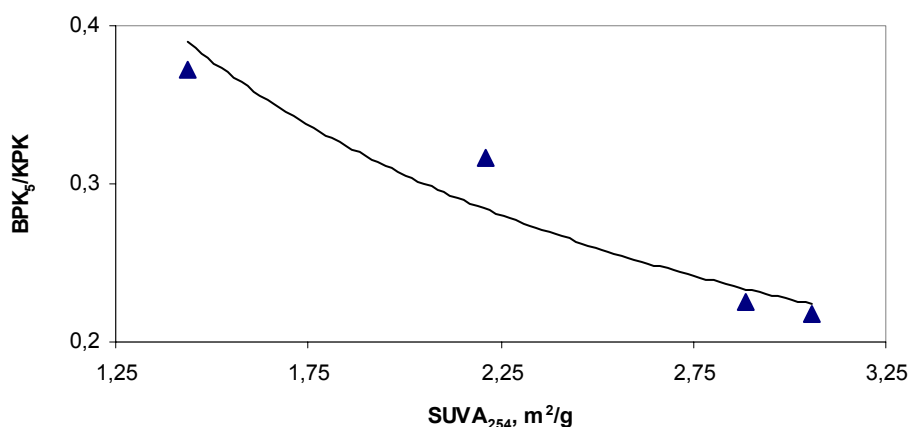
Slika 37. Biorazgradivost produkata ozonizacije u filtriranoj vodi kao funkcija apsorbcije kod 254 nm
