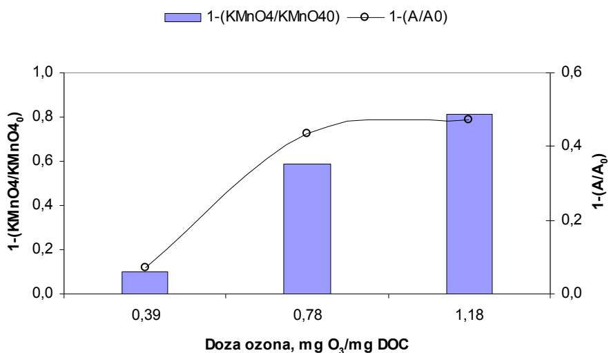
Slika 35. Utjecaj ozonizacije na razgradnju prirodnih organskih tvari u filtriranoj vodi. Redukcija A_{254} i sadržaja organske tvari a , tijekom procesa razgradnje primjenom tri različite doze ozona u protočnom načinu rada b,c,d
