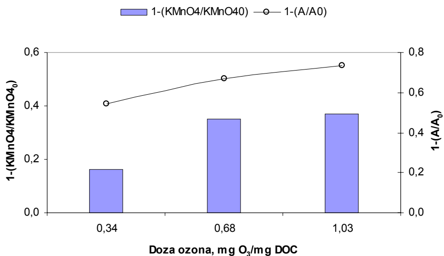
Slika 34. Utjecaj ozonizacije na razgradnju prirodnih organskih tvari u bunarskoj vodi. Redukcija A_{254} i sadržaja organske tvari a , tijekom procesa razgradnje primjenom tri različite doze ozona u protočnom načinu rada b,c,d
