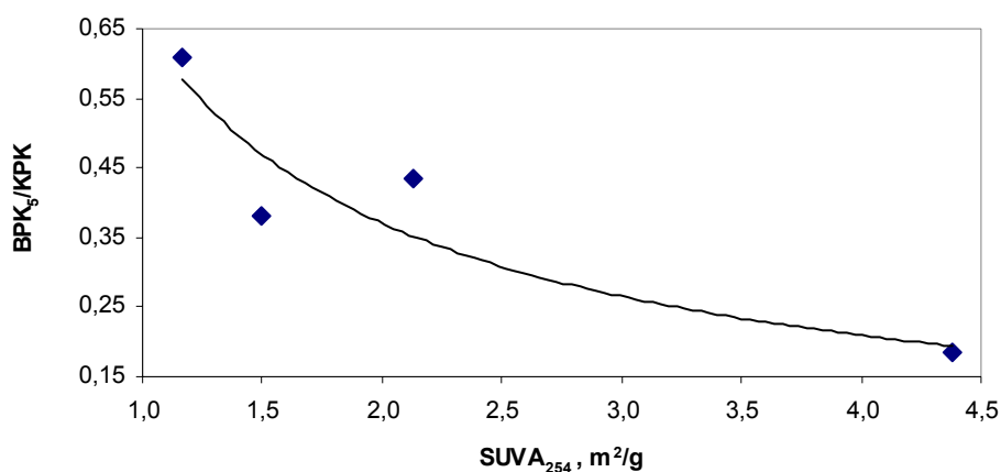
Slika 36. Biorazgradivost produkata ozonizacije u sirovoj bunarskoj vodi kao funkcija apsorbcije kod 254 nm
