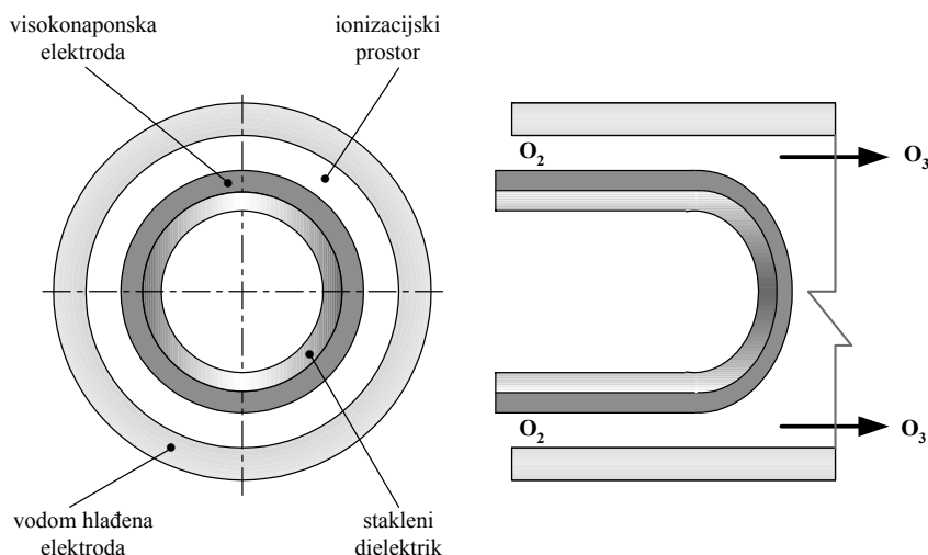
Slika 16. Princip rada tipičnog cijvnog generatora ozona
