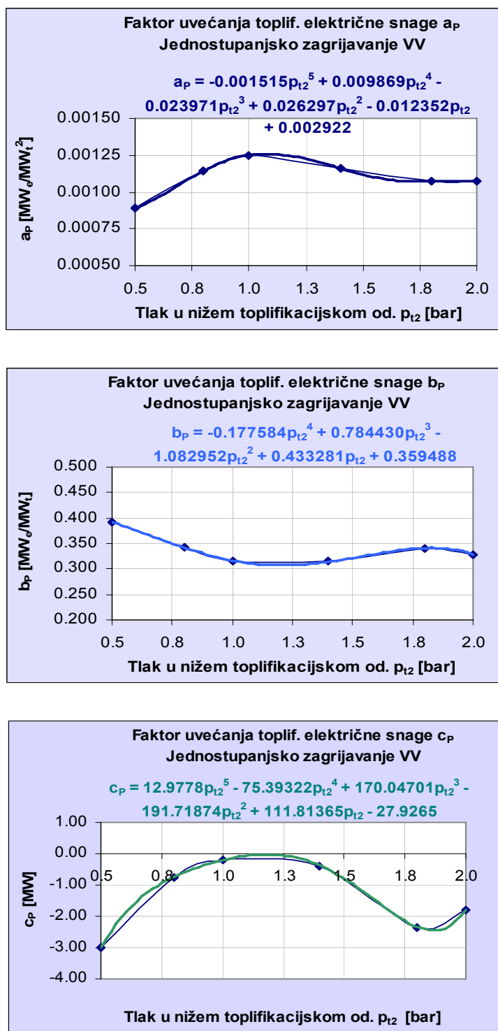
Slika 4.5. Krivulje toplifikacijskog režima rada turbine T-100-130 po toplinskom dijagramu: Funkcionalna zavisnost faktora uvećanja toplifikacijske el. snage o tlaku u nižem toplifikacijskom oduzimanju za jednostupanjsko zagrijavanje
