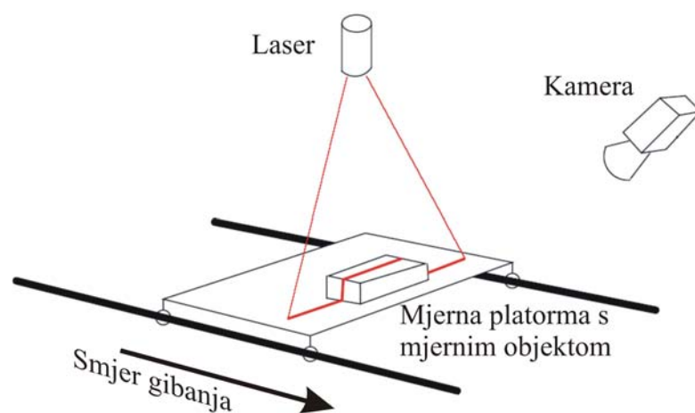
Slika 30. Schematski prikaz postave mjernog senzora
