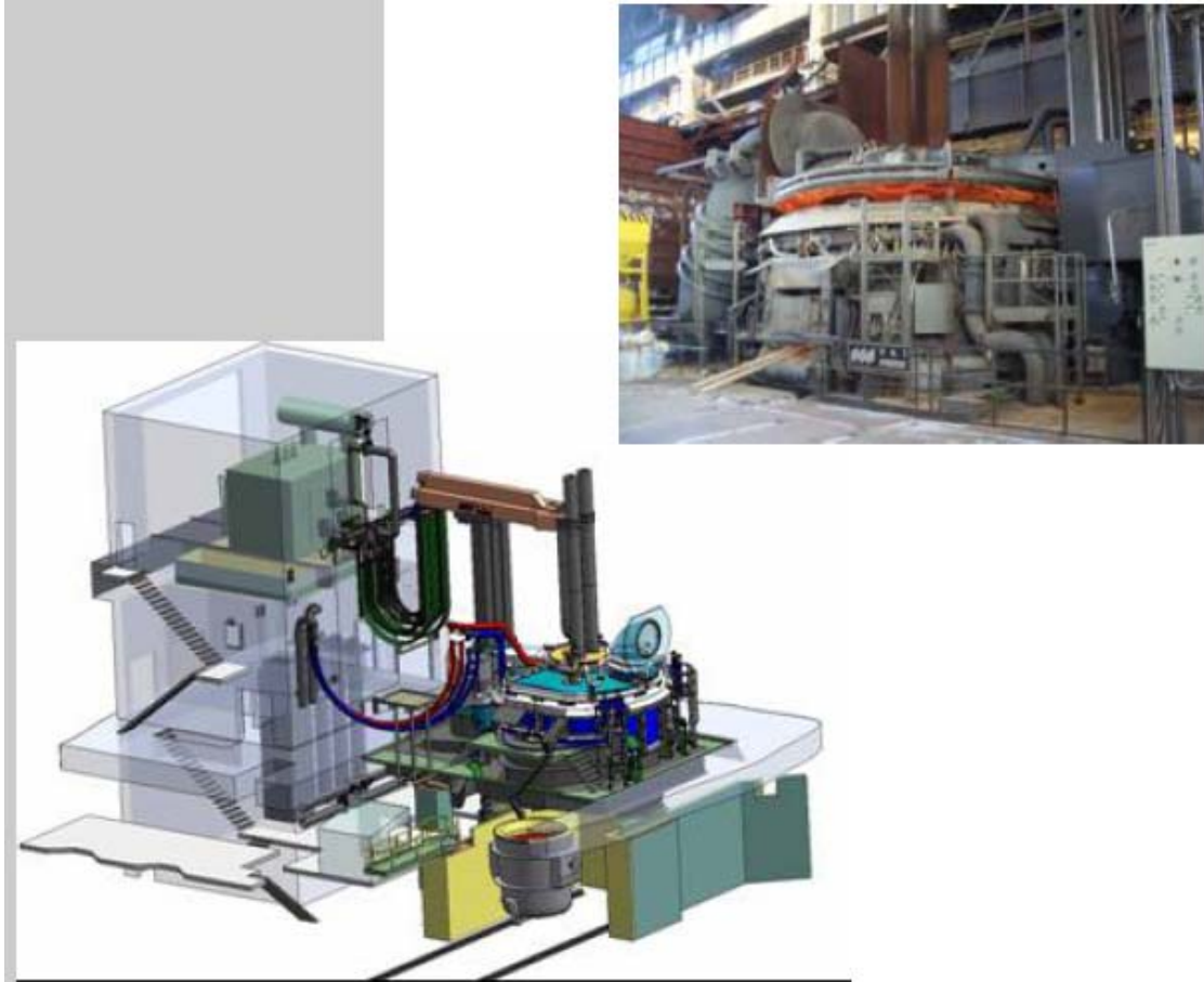
Slika 1-2: Elektroćna peć s pećnim transformatorom
