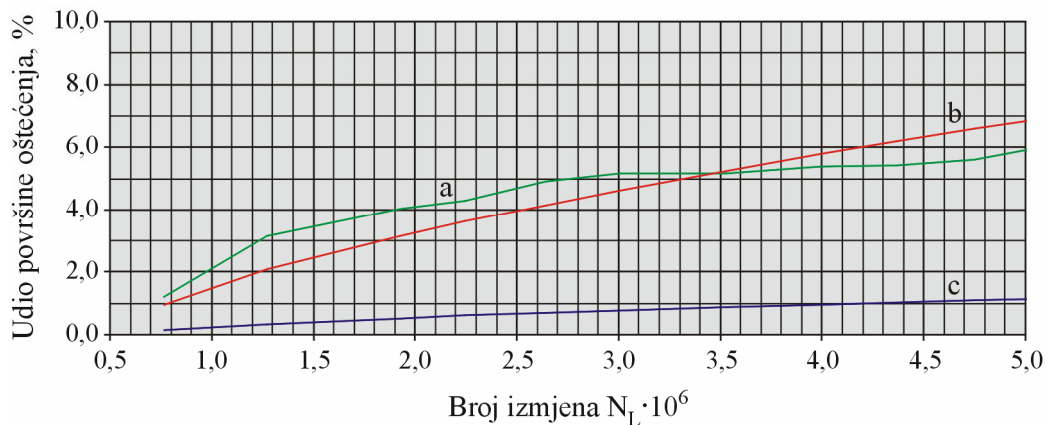
Slika 10.3 Udjeli površine oštećenja za pužno kolo od AlSn6 a) srednja vrijednost udjela površine oštećenja prema površini boka b) udjeli oštećenja prema modelu trošenja dobivenom na temelju pokusa c) udjeli oštećenja prema modelu trošenja iz [4] primijenjenom na nazivni moment iz pokusa
