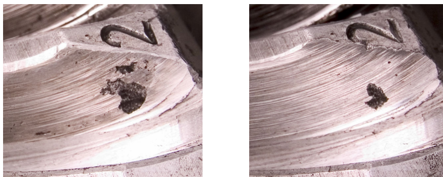
Slika 5.11 Abrazija boka pužnog kola nakon 4,9 \cdot 10^4 ciklusa uslijed nepravilnosti u pogonu (lijevo prije, desno poslije)
