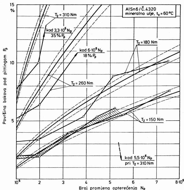
Slika 5.9 Utjecaj opterećenja na povećanje rupičenjem oštećene površine. Brzina klizanja v_k = 2,9 \text{ m/s} je konstanta.
