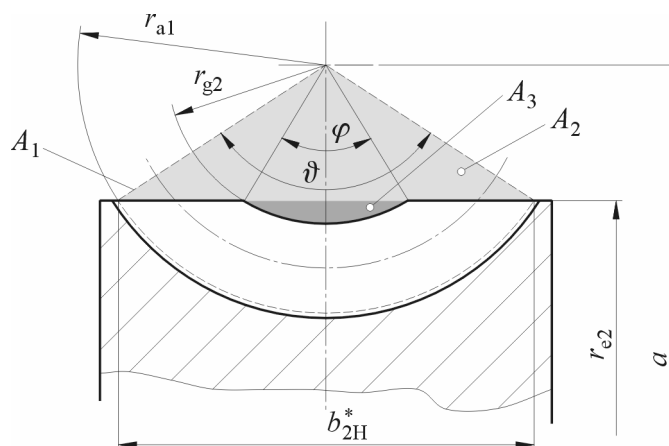
Slika 7.3 Definiciranje parcijalnih površina pomoću dimenzija pužnog para
