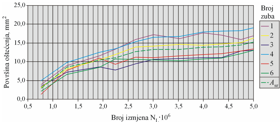
Slika 10.2 Površine oštećenja u zavisnosti od broja ciklusa za pužno kolo od AlSn6
