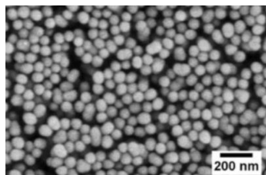
Slika 4-3 SEM snimka mozoporoznih \text{SiO}_2 čestica [104]
