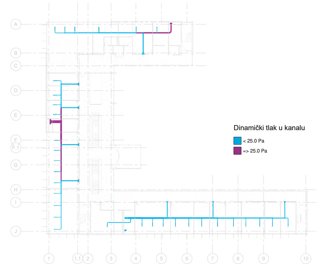
3 Dobavni sustav 1 : 200
