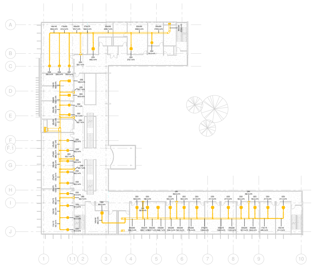
1 Odsisni sustav 1 : 200
