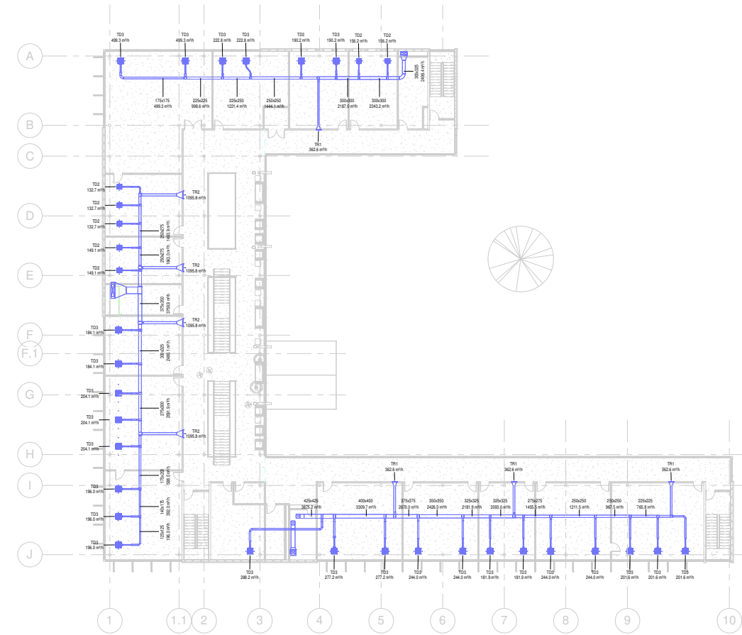
2 Dobavni sustav 1 : 200
