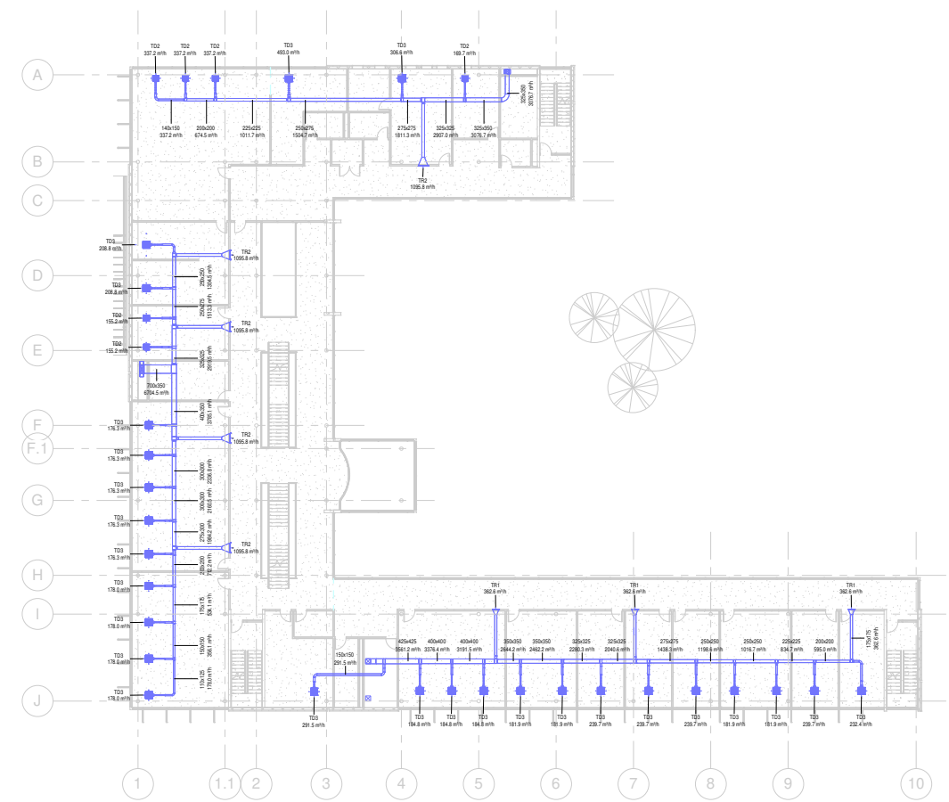
2 Dobavni sustav 1 : 200
