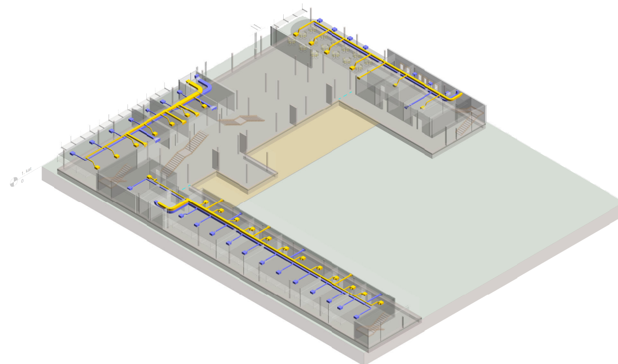
3 Izometrija kata
