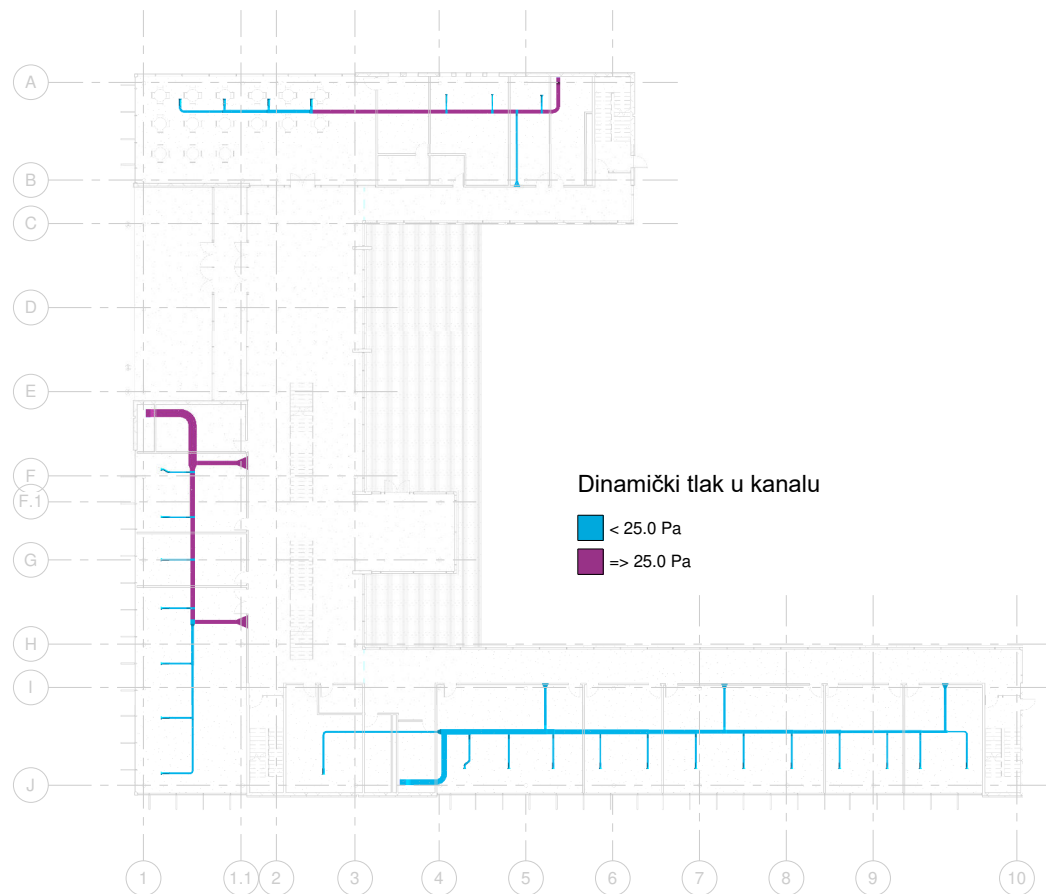
3 Dobavni sustav 1 : 200
