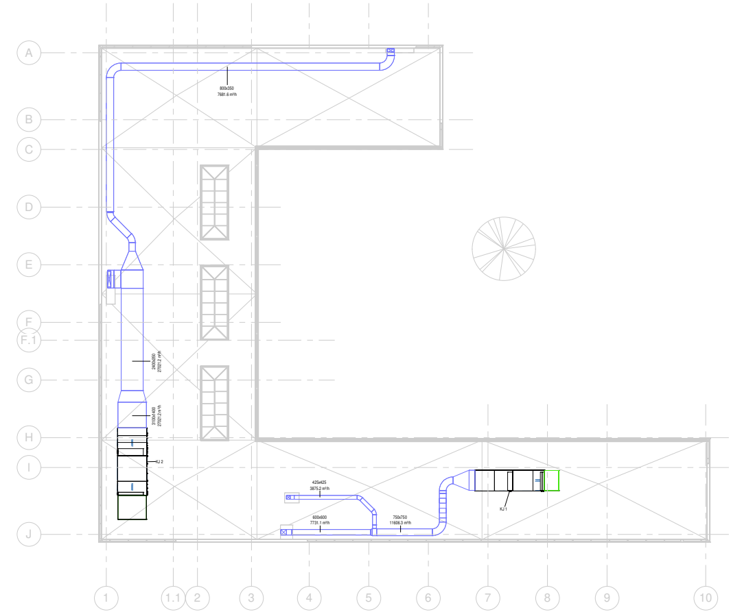
2 Dobavni sustav 1 : 200
