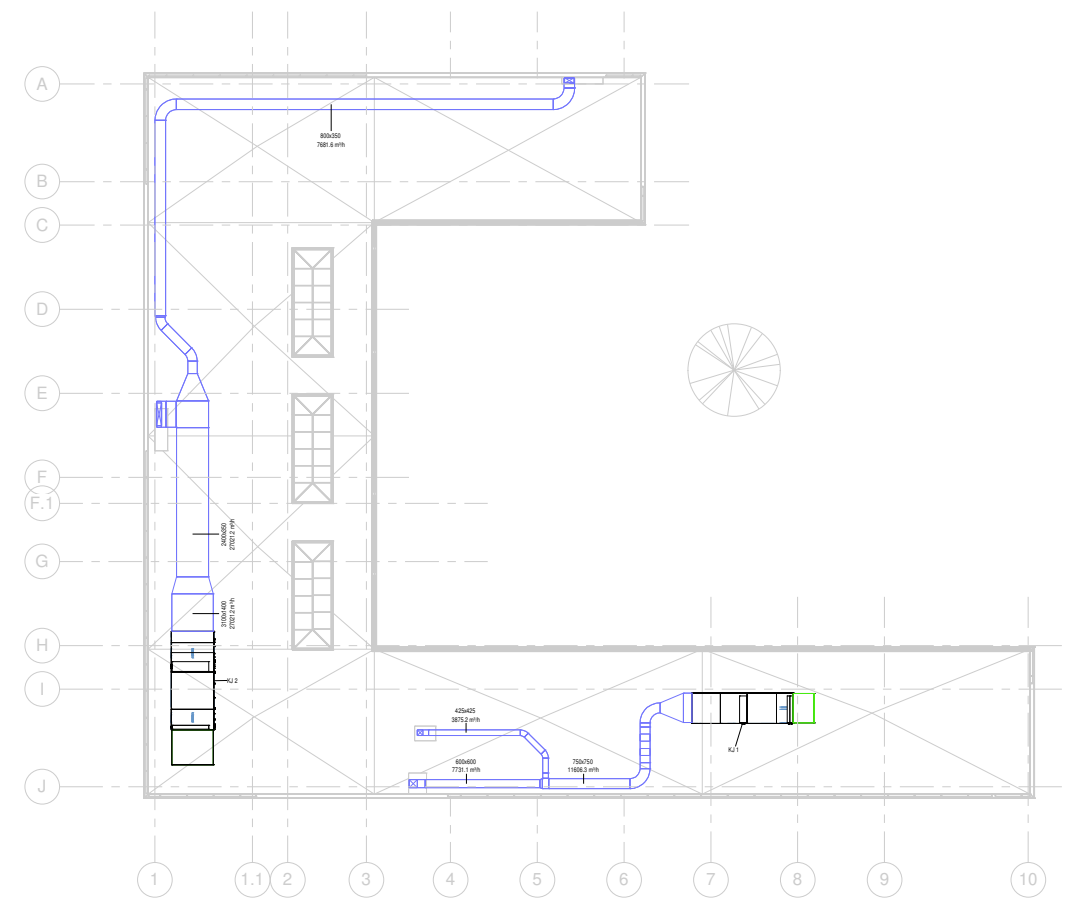
2 Dobavni sustav 1 : 200
