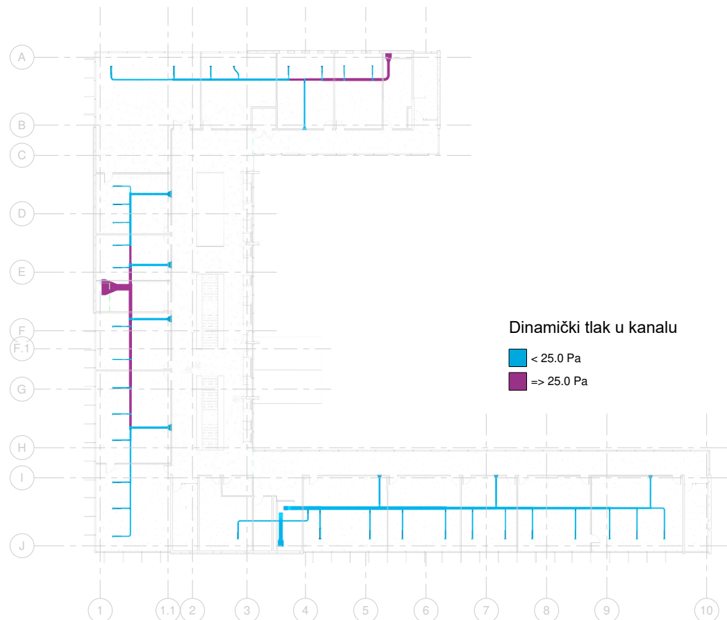
3 Dobavni sustav 1 : 200
