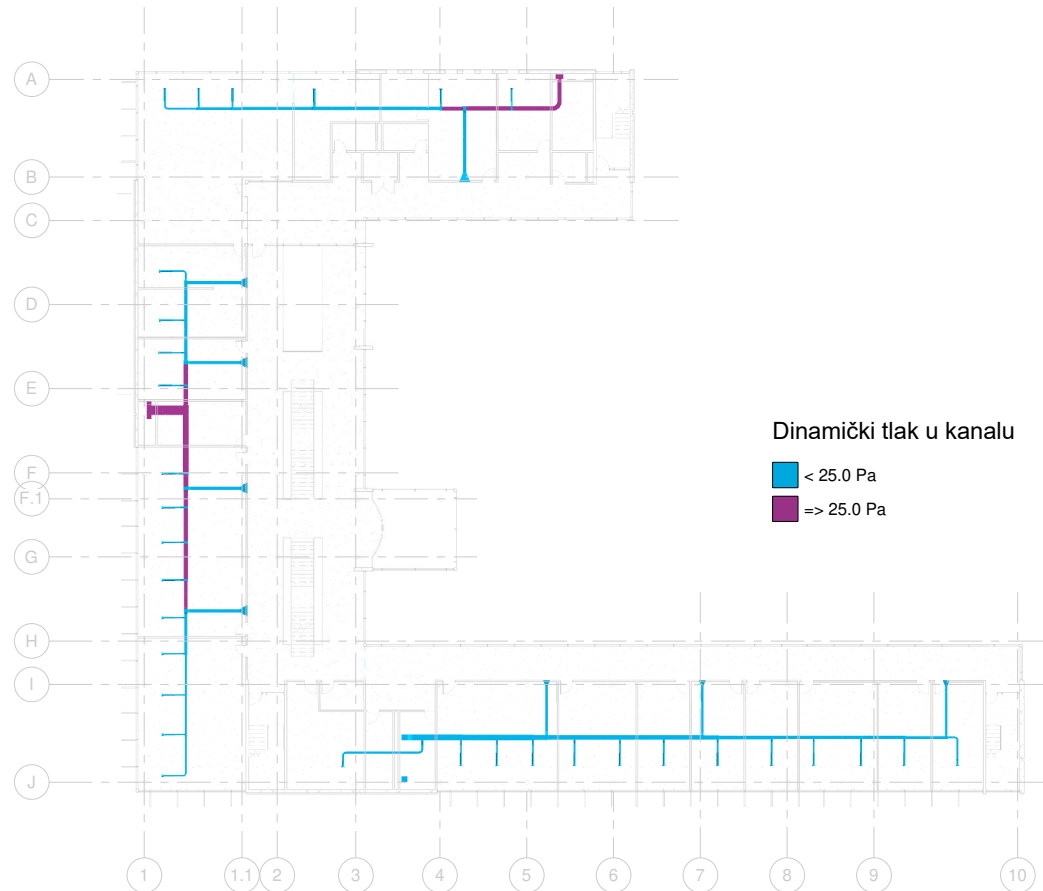
3 Dobavni sustav 1 : 200
