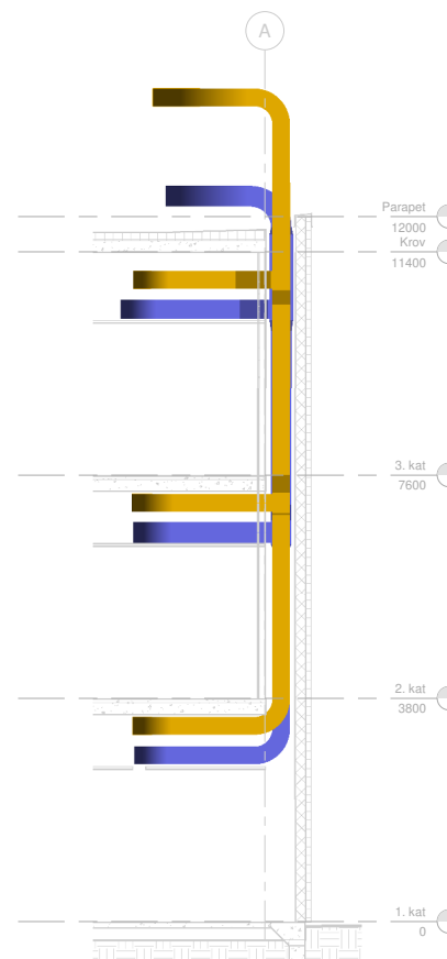
③ V_VO_3 1 : 50
