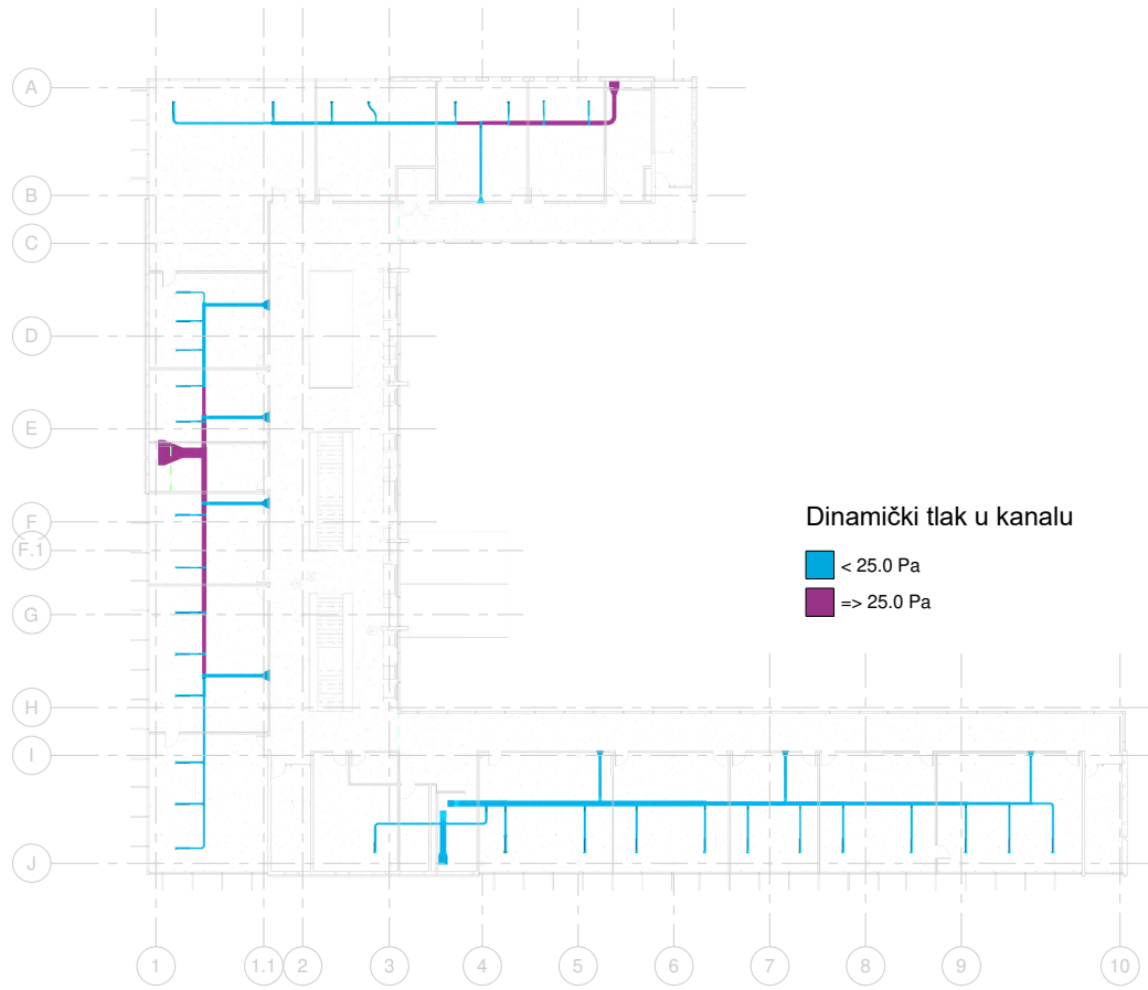
3 Dobavni sustav 1 : 200
