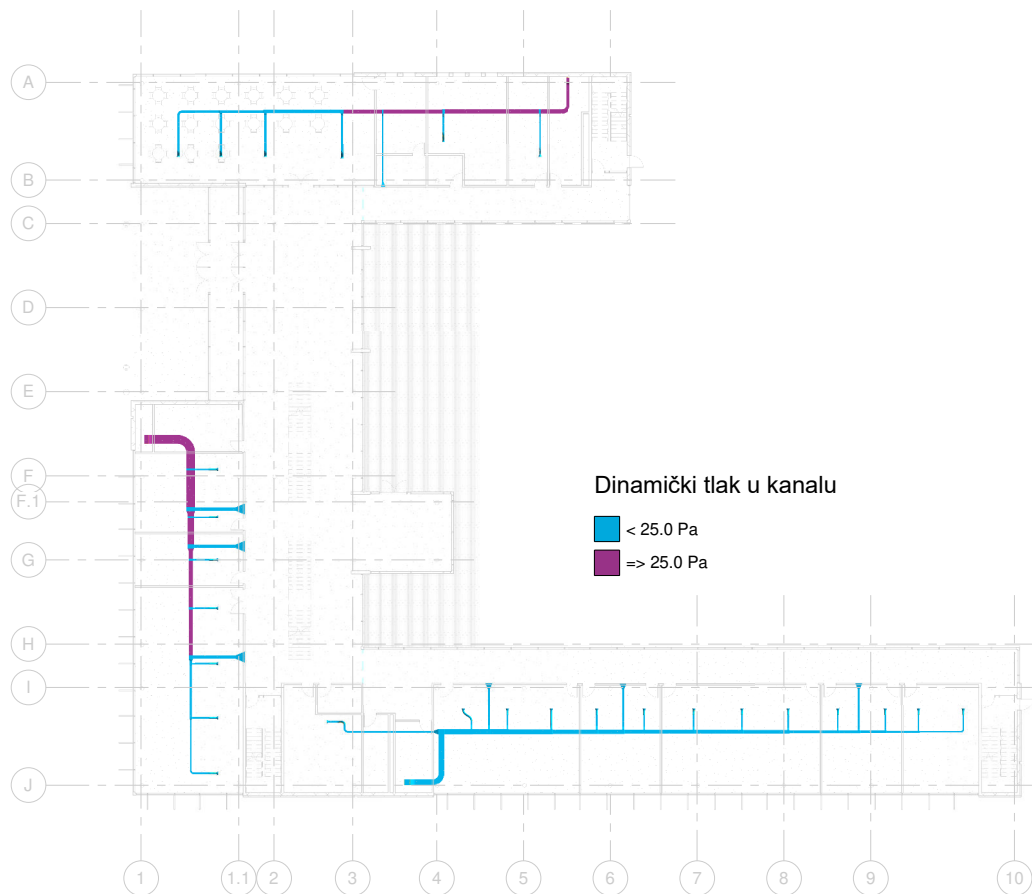
4 Odsisni sustav 1 : 200
