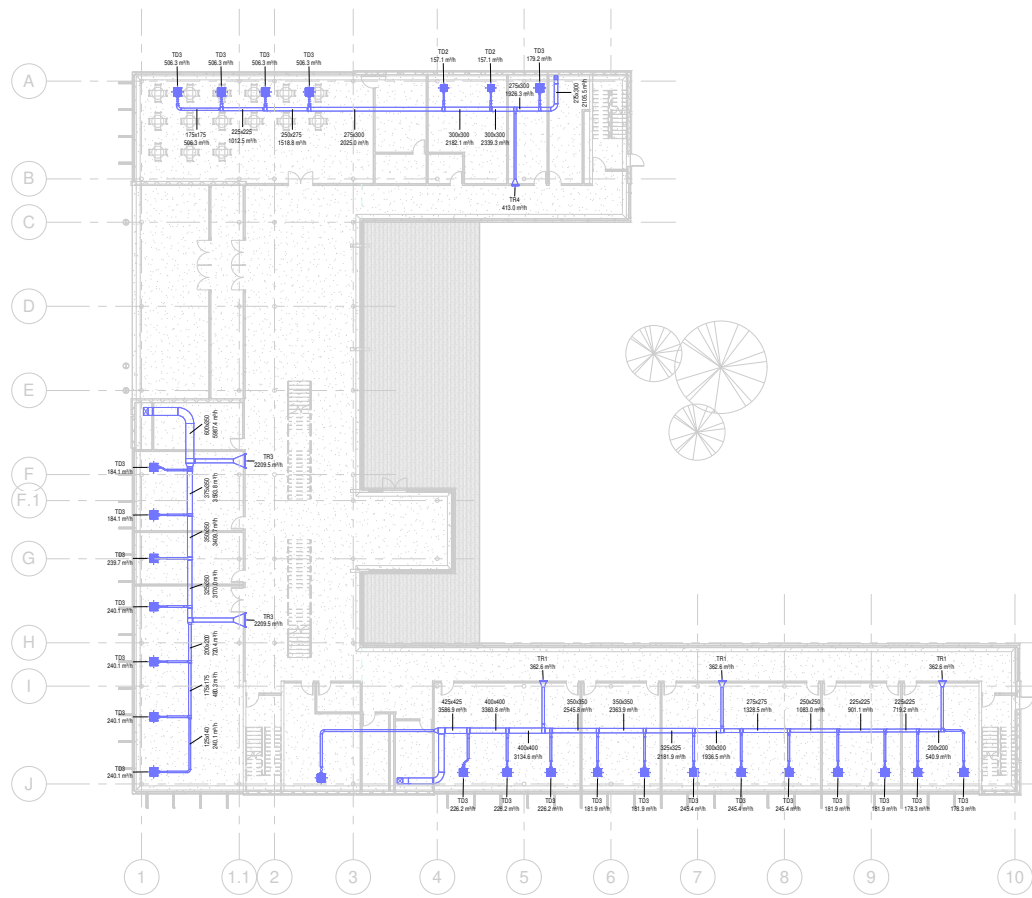
1 Dobavni sustav 1 : 200
