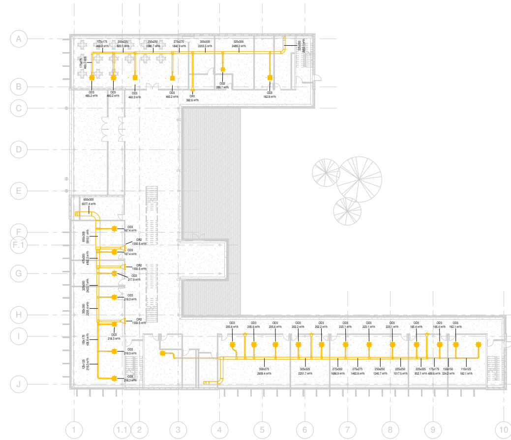
2 Odsisni sustav 1 : 200
