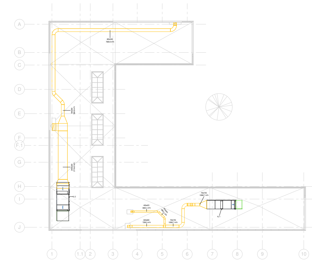
1 Odsisni sustav 1 : 200
