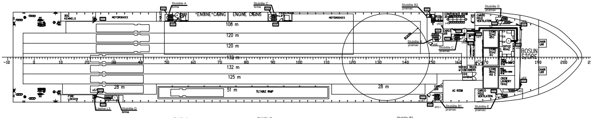
PALUBA 8 14700mm od BL
