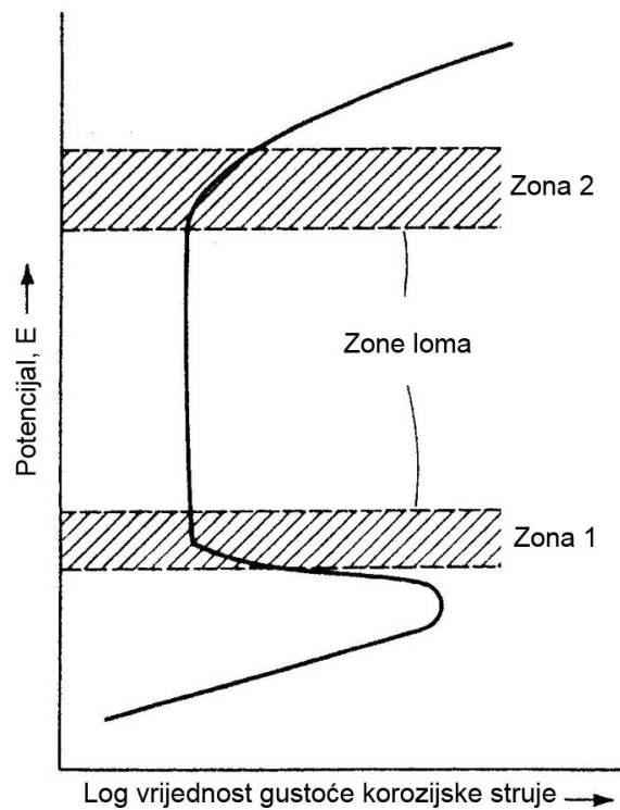
Slika 12: Utjecaj elektrodnog potencijala na osjetljivost prema napetnosnoj koroziji [11]
