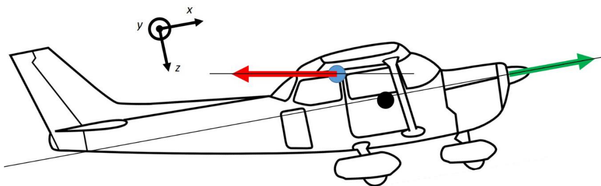
Slika 6 Shematski prikaz vektora sile otpora i pogonske sile za motor s nulnim postavnim kutom
