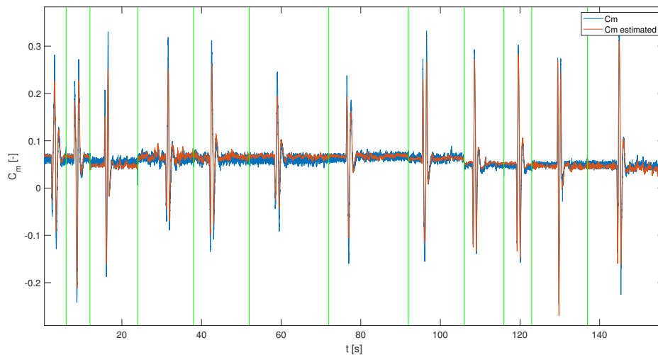
Slika 0.7: Linearne regresije koeficijenta momenta propinjanja za niz kratkotrajnih manevara
