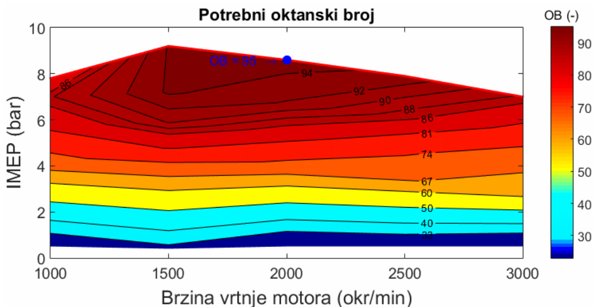
Slika 33. Topografski dijagram potrebnog oktanskog broja
