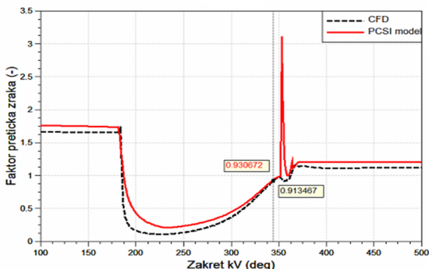
Slika 23. Usporedba faktora pretička zraka u pretkomori
