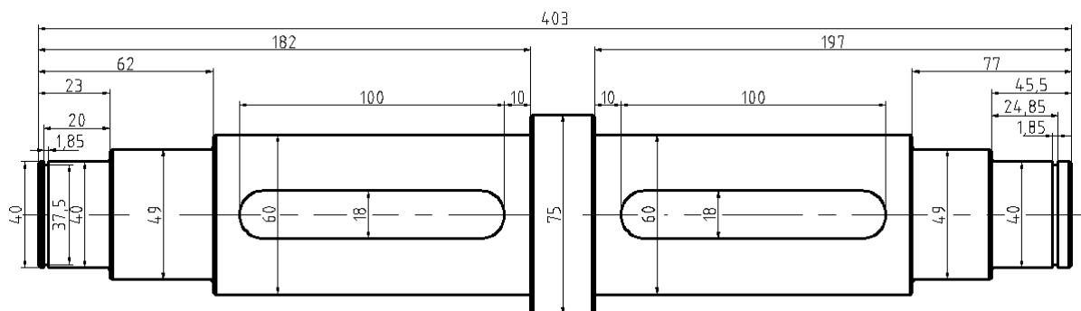
Slika 44: Dimenzije analiziranog vratila
