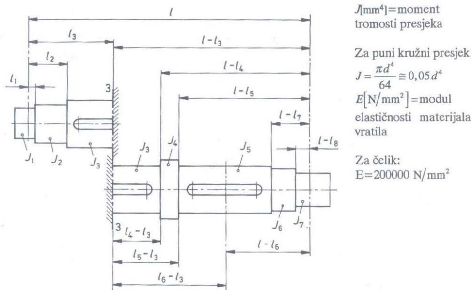
Slika 42: Ukliještenje na mjestu 3.
