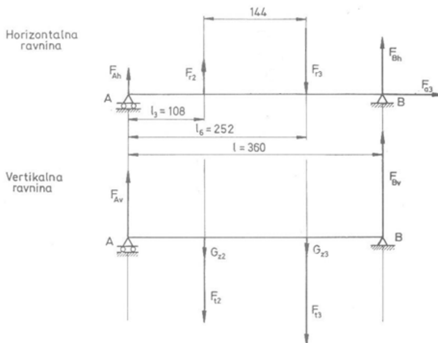
Slika 41: Opterećenja na vratilo
