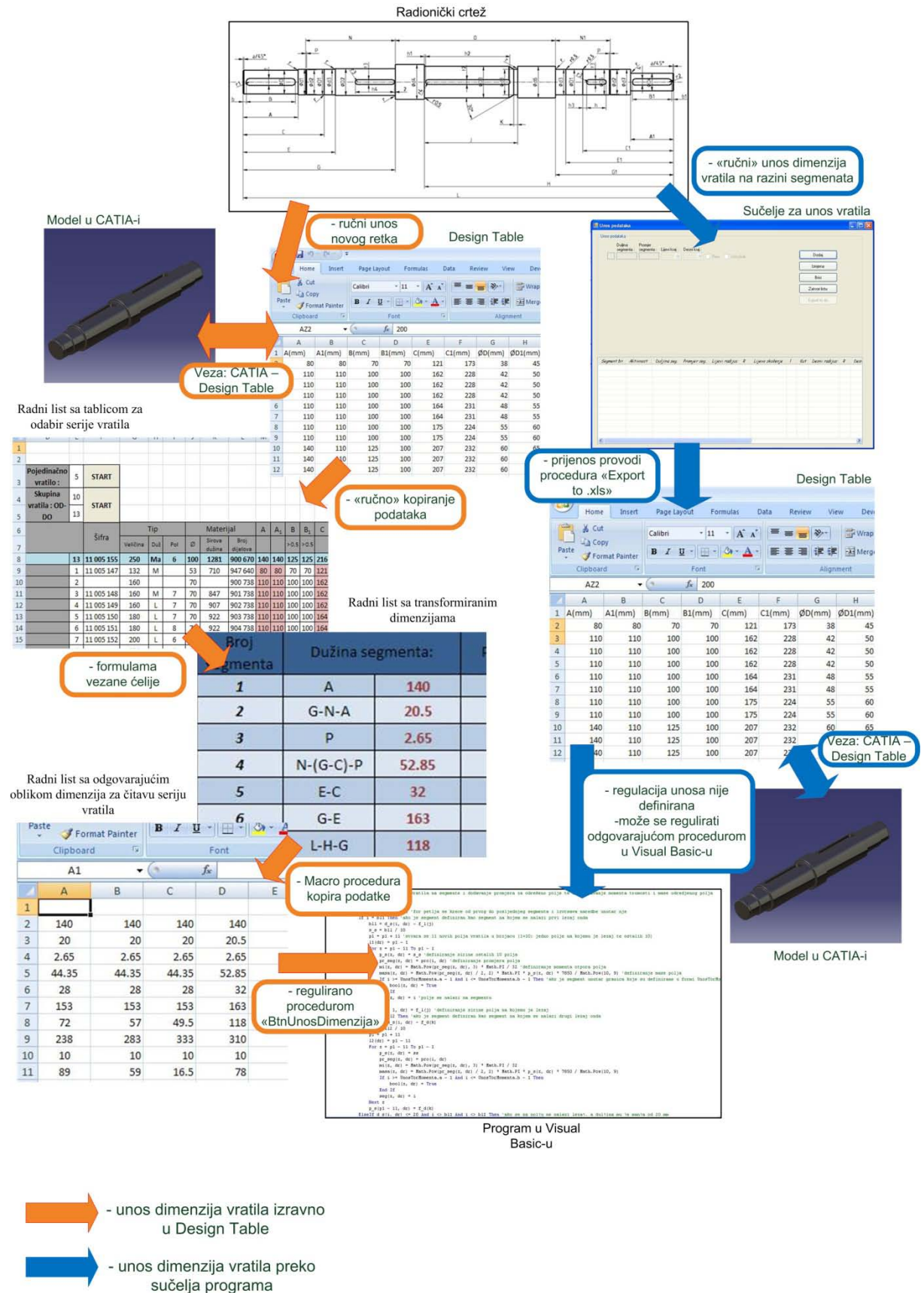
Slika 1: Unos i transformacija dimenzija vratila
