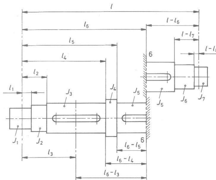
Slika 43: Uklještenje na mjestu 6.
