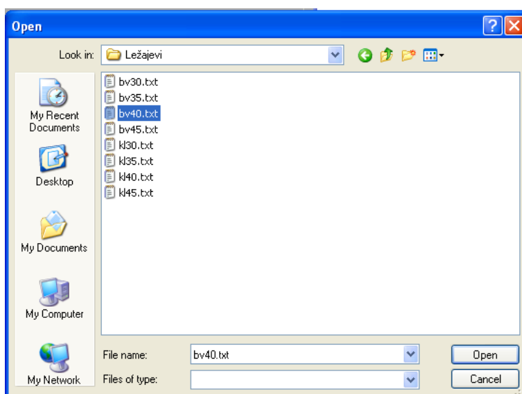
Slika 20: Open Dialog
