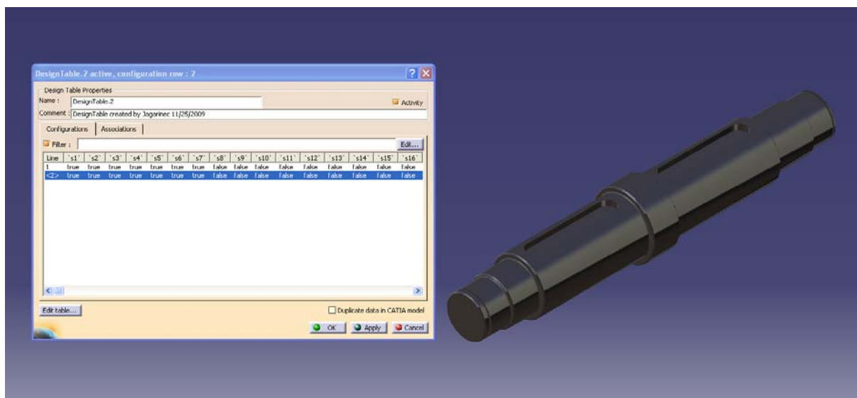
Slika 8 : Model vratila i Design Table u CATIA-i
